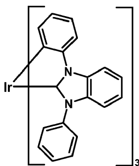
Ir(DPBIC) 3
