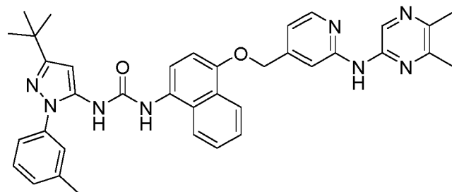
1-(3-( tert -butyl)-1-( m -tolyl)-1 H -pyrazol-5-yl)-3-(4-((2-((5,6-dimethylpyrazin-2-yl)amino)pyridin-4-yl)methoxy)naphthalen-1-yl)urea.
