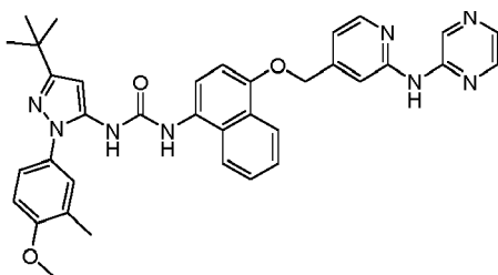
1-(3-( tert -butyl)-1-(4-methoxy-3-methylphenyl)-1 H -pyrazol-5-yl)- 3-(4-((2-(pyrazin-2-ylamino)pyridin-4-yl)methoxy)naphthalen-1-yl)urea
