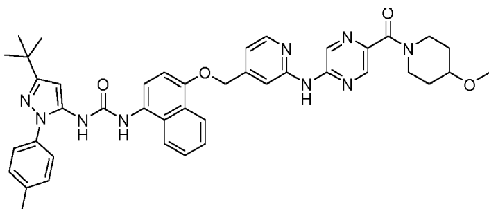
1-(3-( tert -butyl)-1-( p -tolyl)-1 H -pyrazol-5-yl)-3-(4-((2-((5-(4-methoxypiperidine-1-carbonyl)pyrazin-2-yl)amino)pyridin-4-yl)methoxy)naphthalen-1-yl)urea
