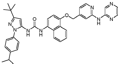
1-(3-( tert -butyl)-1-(4-isopropylphenyl)-1 H -pyrazol-5-yl)- 3-(4-((2-(pyrazin-2-ylamino)pyridin-4-yl)methoxy)naphthalen-1-yl)urea
