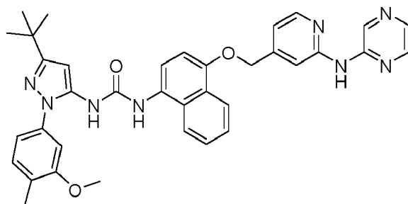
1-(3-( tert -butyl)-1-(3-methoxy-4-methylphenyl)-1 H -pyrazol-5-yl)-3-(4-((2-(pyrazin-2-ylamino)pyridin-4-yl)methoxy)naphthalen-1-yl)urea.
