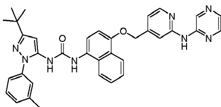
1-(3-( tert -butyl)-1-( m -tolyl)-1 H -pyrazol-5-yl)-3-(4-((2-(pyrazin-2-ylamino)pyridin-4-yl)methoxy)naphthalen-1-yl)urea
