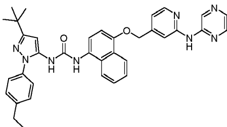
1-(3-( tert -butyl)-1-(4-ethylphenyl)-1 H -pyrazol-5-yl)-3-(4-((2-(pyrazin-2-ylamino)pyridin-4-yl)methoxy)naphthalen-1-yl)urea
