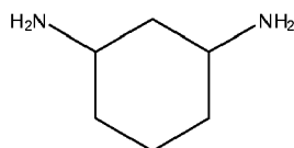
Cyclohexane-1,3-diamine,
