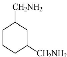
1, 3-bis(methylamine)-cyclohexane,
