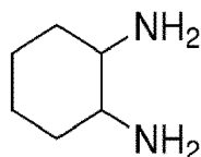
Cyclohexane-1,2-diamine
