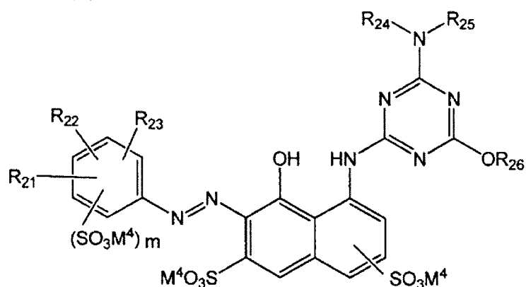
Formula (D)
