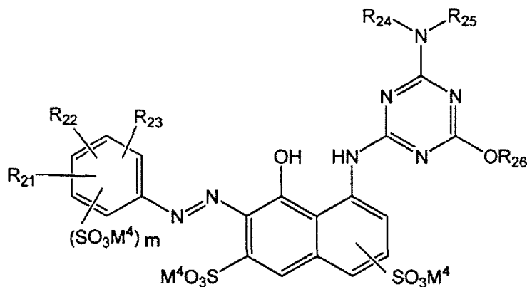
Formula (D)
