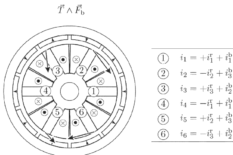
Fig. 2d i_1 = 0, i_2 = -168 \text{ A}, i_3 = 0, i_4 = 0, i_5 = 0, i_6 = 168 \text{ A}
