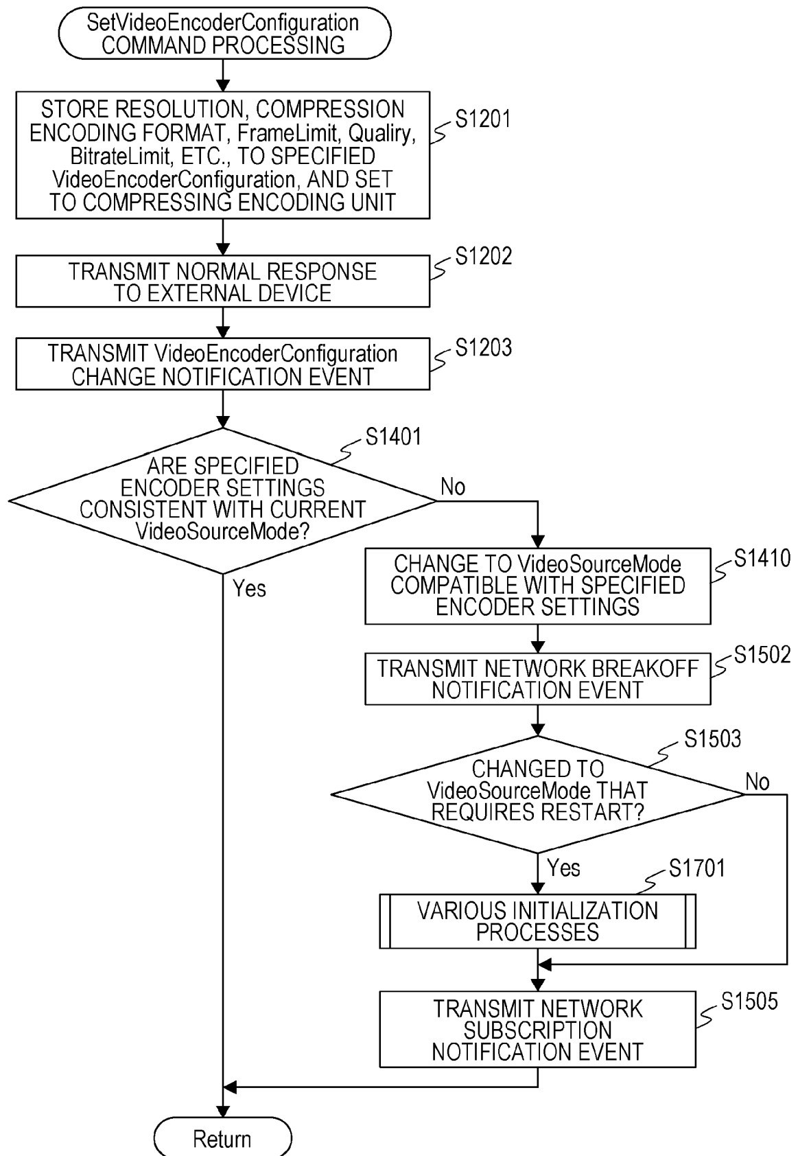
FIG. 20
