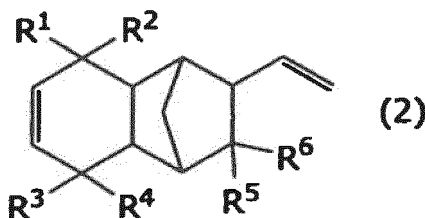
[Chem. 3]
