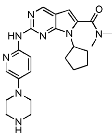
Ribociclib
