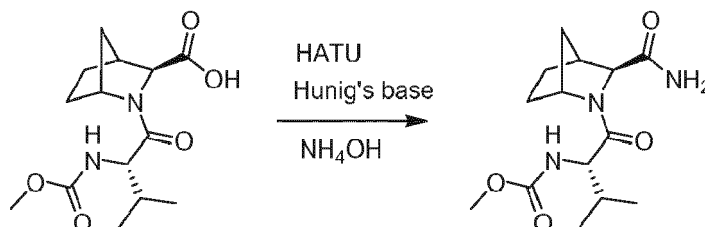
methyl (2S)-1-((3S)-3-carbamoyl-2-azabicyclo[2.2.1]heptan-2-yl)-3-methyl-1-oxobutan-2-ylcarbamate
