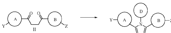
Scheme VI
