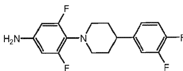
4-(4-(3,4-difluorophenyl)piperidin-1-yl)-3,5-difluoroaniline
