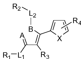
Formula (D);
