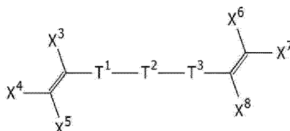
EWG 1 -T 1 -T 2 -T 3 -EWG 2
