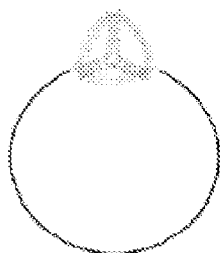
Full M13mp18
