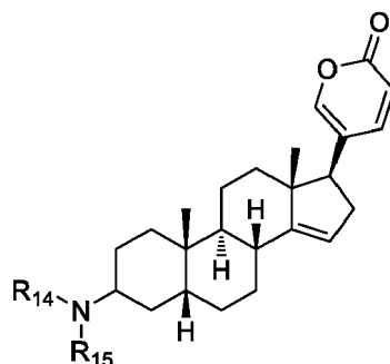
Formula Ik
