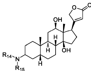
Formula li
