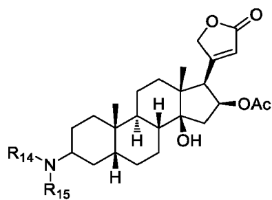
Formula lj
