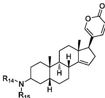
Formula Ik
