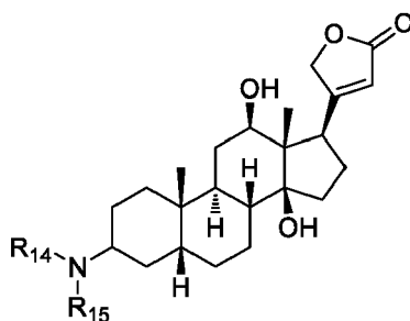
Formula li
