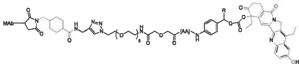
MAb-CLX-SN-38,
