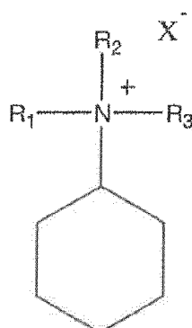
[Chem. 3]
