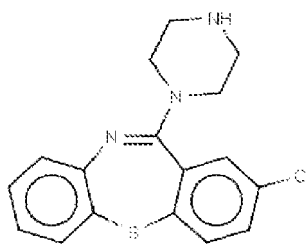
(2-Cl-norQTP)
