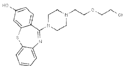
(7-OH-QTP)
