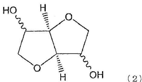
[Chem. 6]
