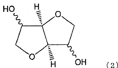
[Chem. 3]
