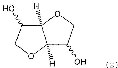
[Chem. 3]
