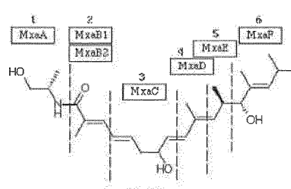
Myxalamat S
