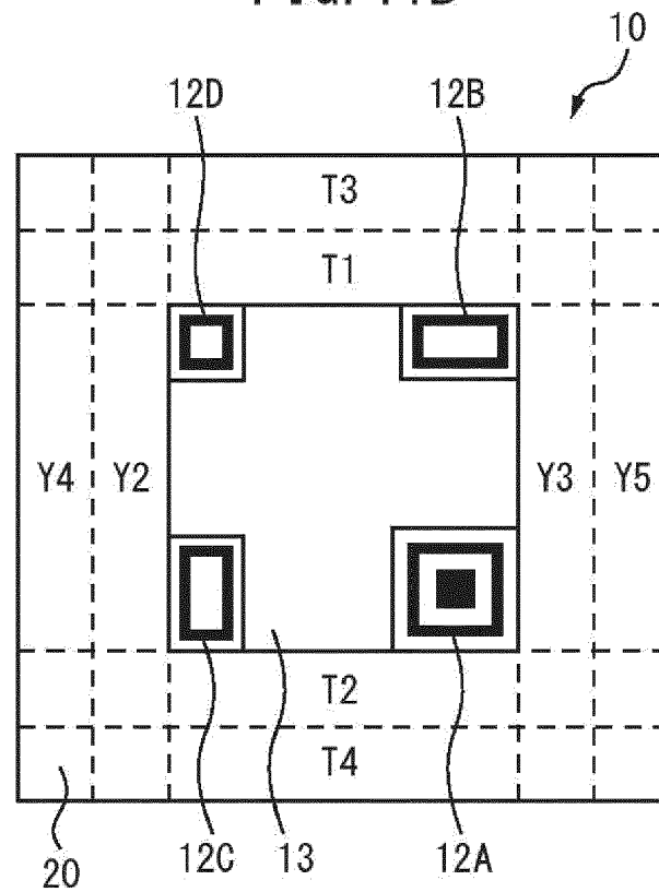
FIG. 11B
