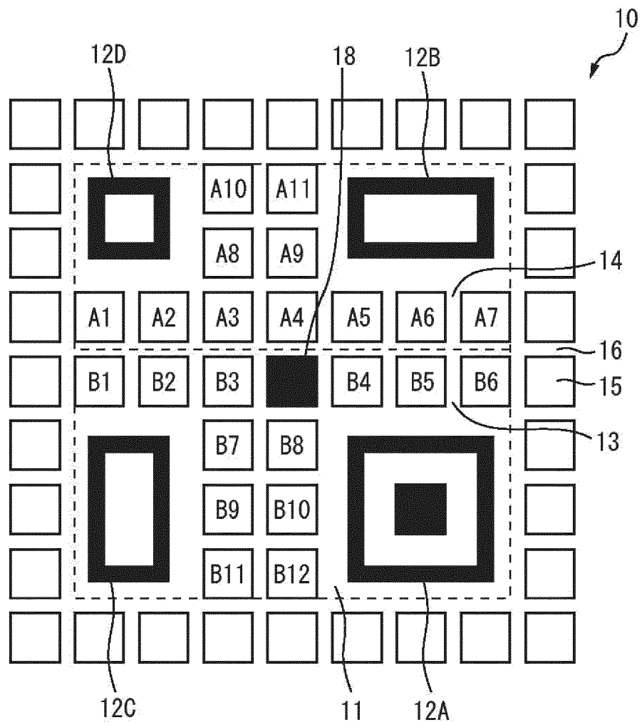
FIG. 12A
