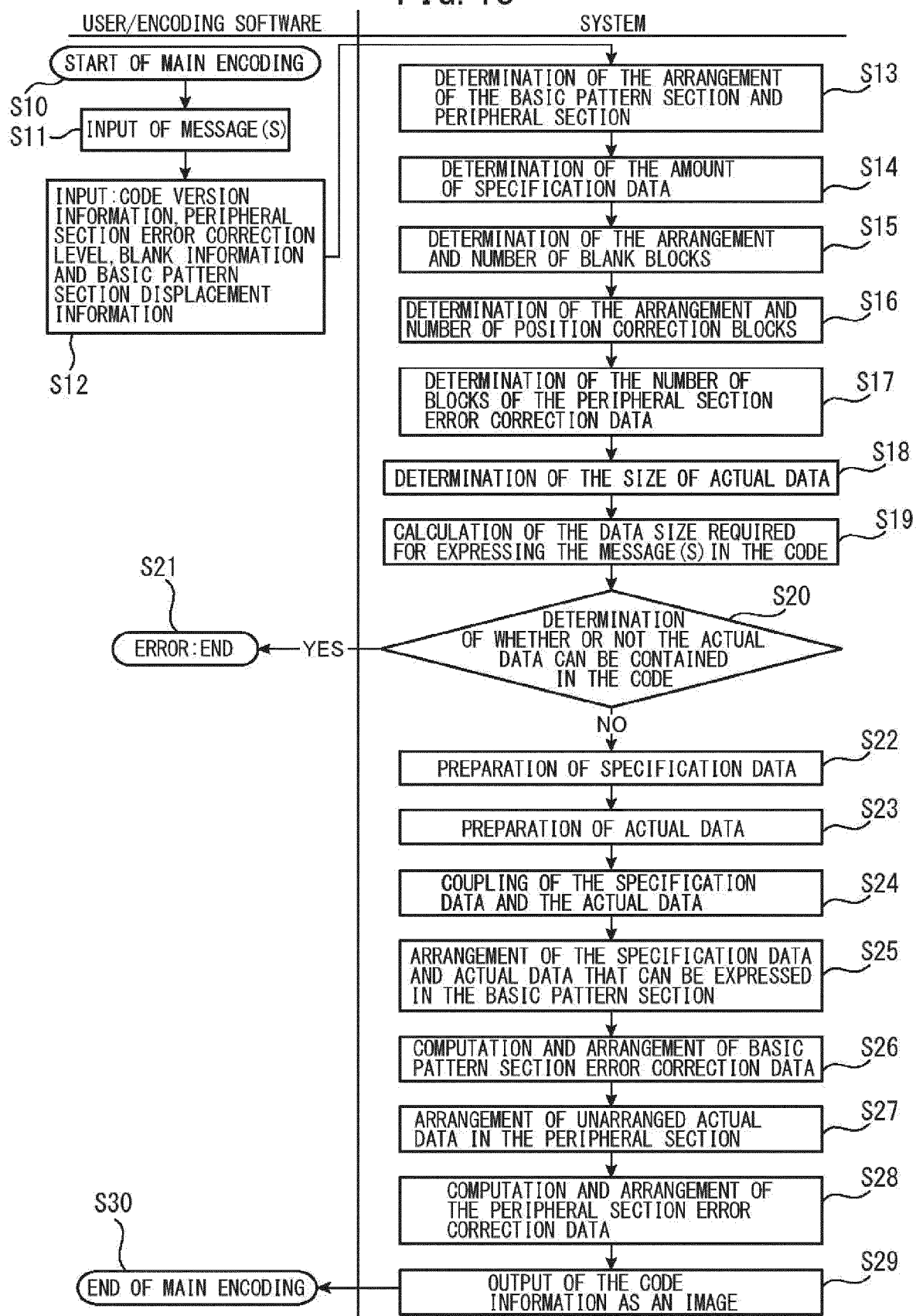
FIG. 18
