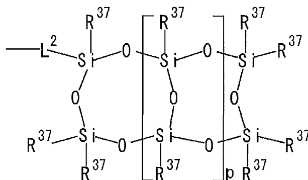
[Chem. 23]
