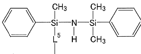
[Chem. 45]
