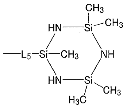
[Chem. 45]
