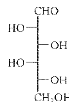
D-Idose (D-Ido)
