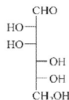
D-Mannose (D-Man)
