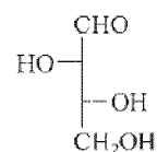
D-Threose
