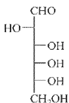
D-Altrose (D-Alt)
