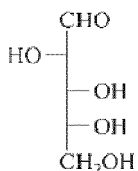
D-Arabinose (D-Ara)
