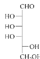
D-Talose (D-Tal)
