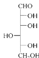
D-Gulose (D-Gul)
