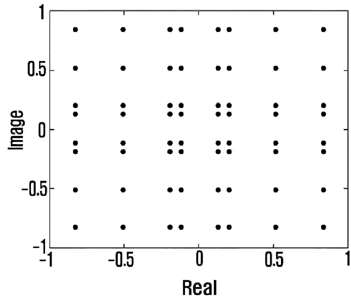
(d) PC4: Rank2(QPSK+16QAM)
