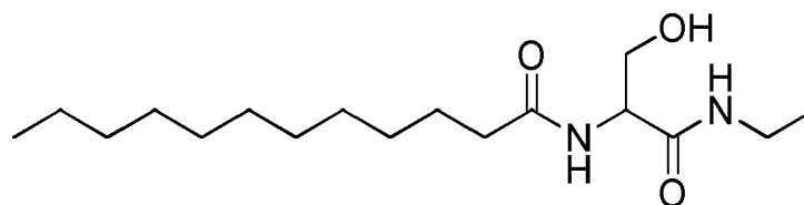
N-(1-(ethylamino)-3-hydroxy-1-oxopropan-2-yl)dodecanamide
