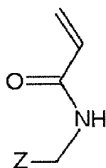
(IX),
