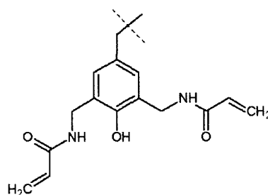
(II'b).
