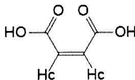
Maleic acid:
