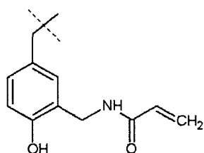
(II'a)
