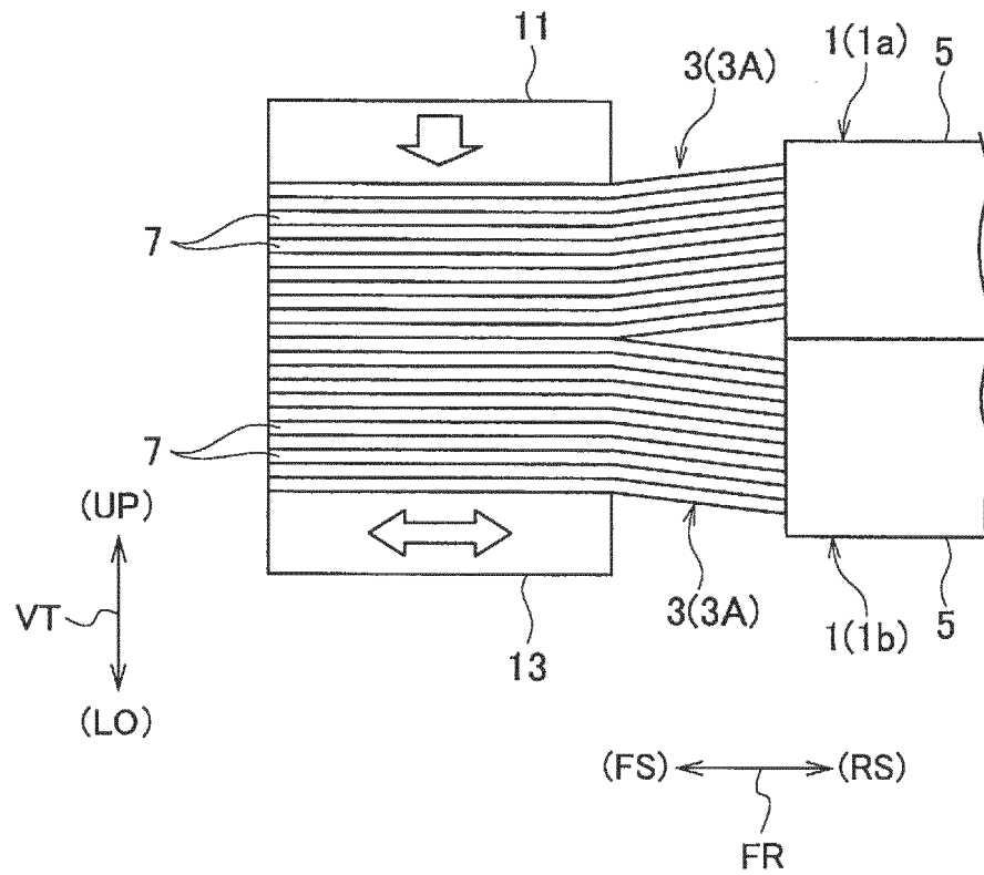
FIG. 8A
