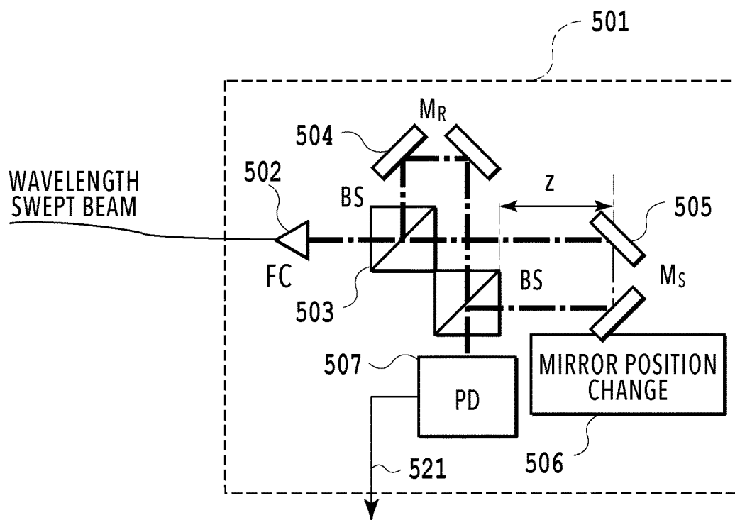
FIG.9D
