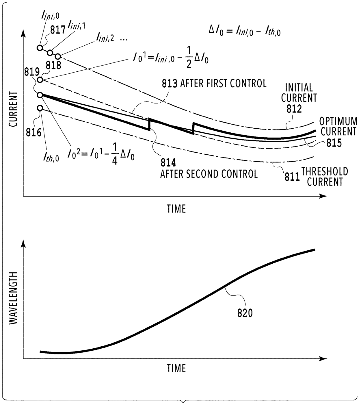
FIG.14
