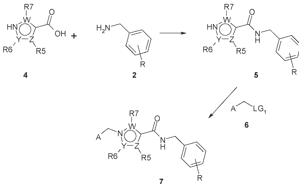
Scheme 2a
