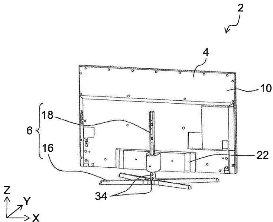
FIG. 13H
