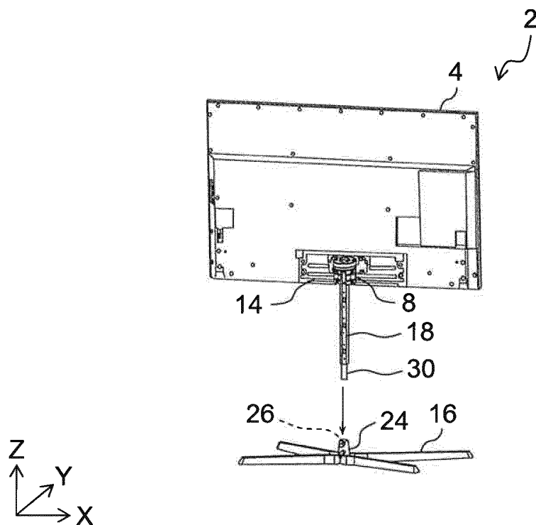
FIG. 12C
