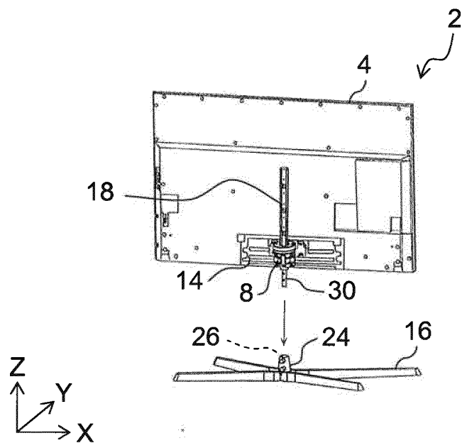
FIG. 13G
