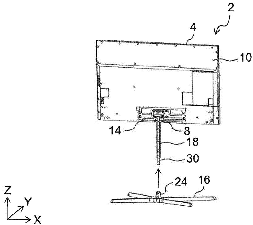
FIG. 13A
