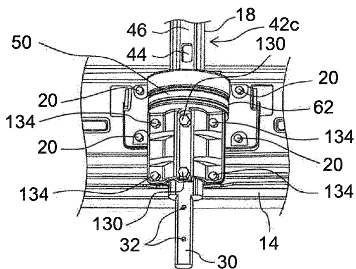
FIG. 13F
