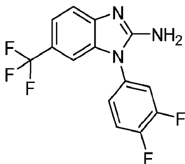
1-(3-fluoro-4-(trifluoromethoxy)phenyl)-6-(trifluoromethyl)-1H-benzo[d]imidazol-2-amine
