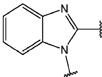
benzoimidazol-1,2-yl
