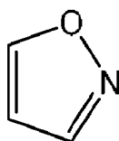
isoxazolyl
