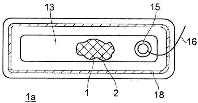
FIG. 3b/plan
