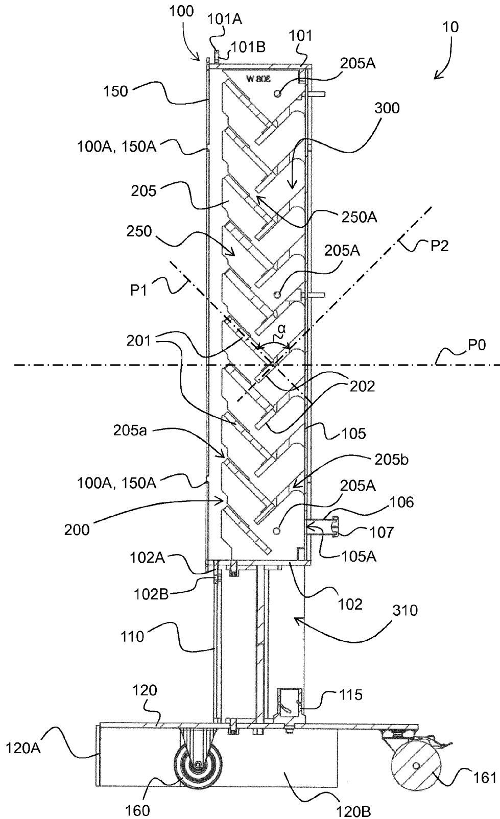
Fig. 5B (C-C)
