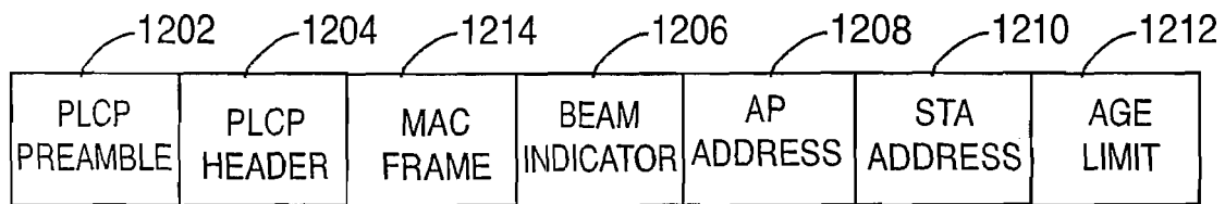
1220 FIG. 12b
