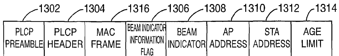
1320 FIG. 13b
