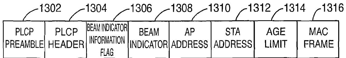
1300 FIG. 13a
