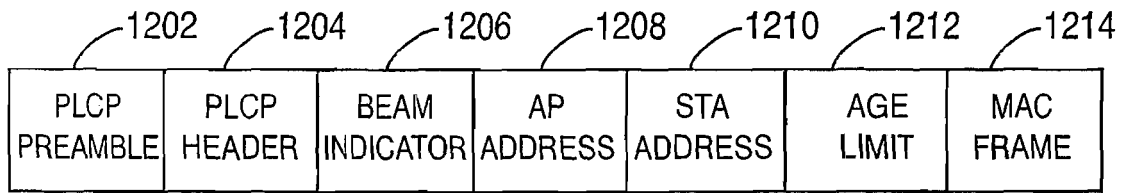
1200 FIG. 12a
