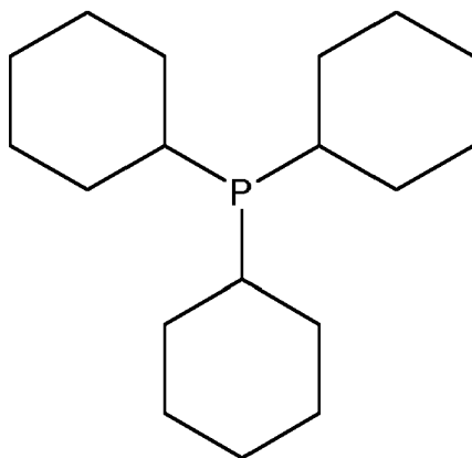
(3) (Vergleichsverbindung)
