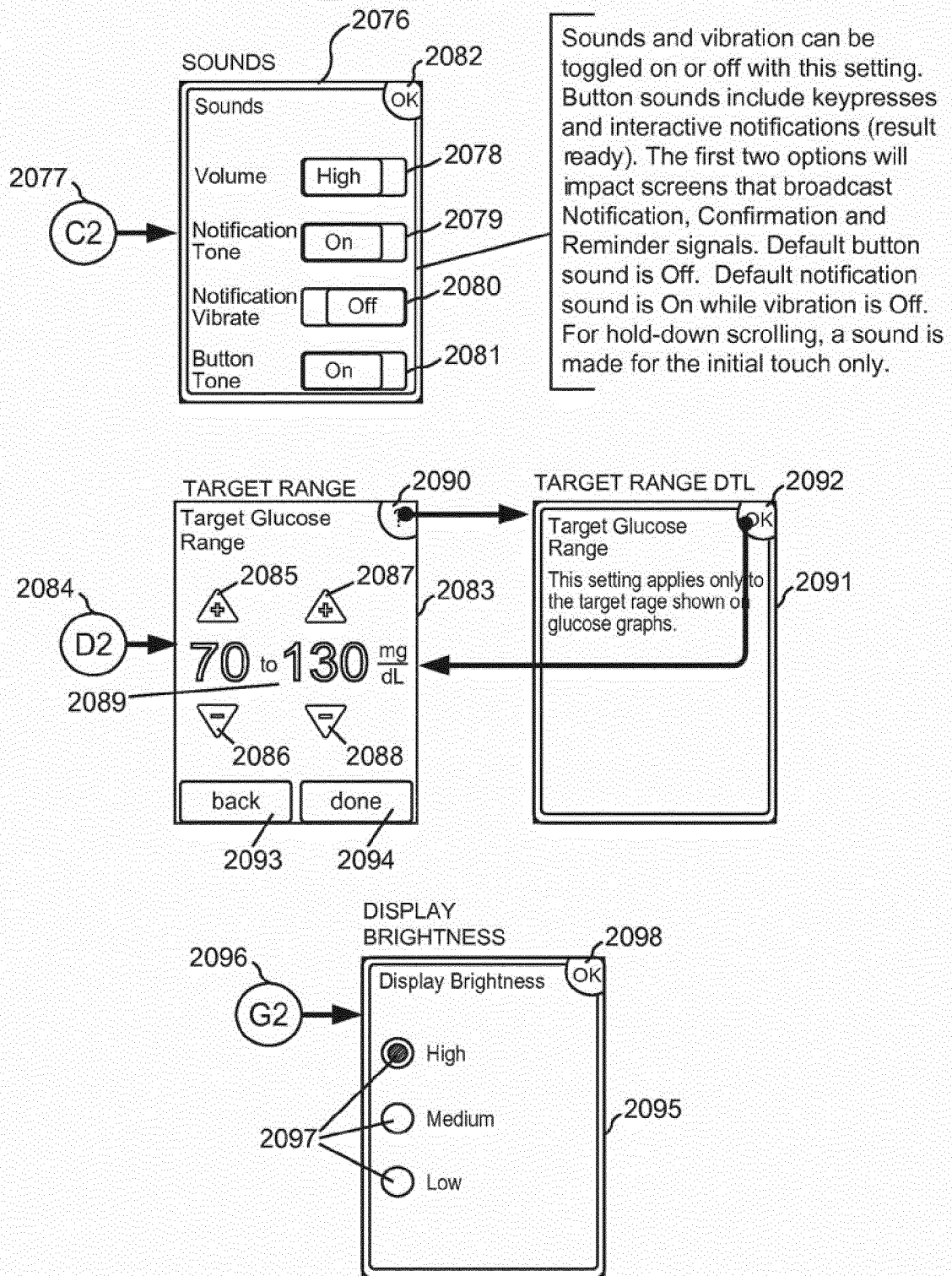
FIG. 25 (Cont)
