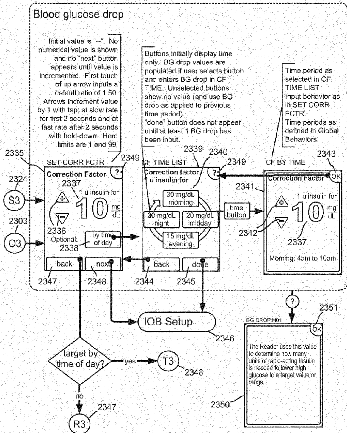
FIG. 32 (Cont)
