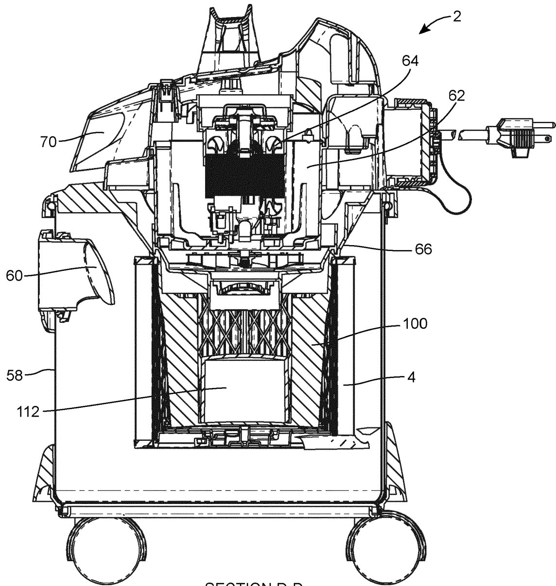
SECTION D-D
