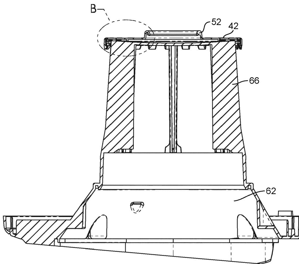
SECTION A-A FIG. 15B
