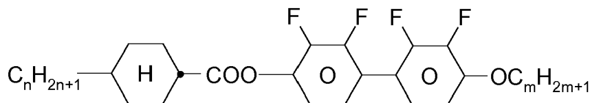
CZYY-n-Om
