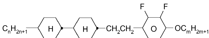
CCEY-n-Om
