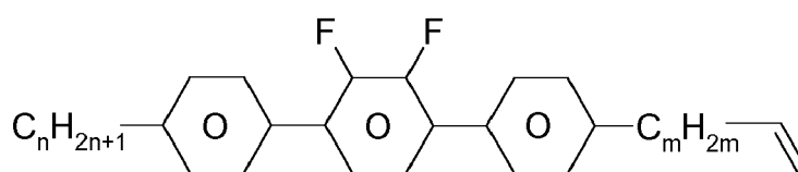
PYP-n-mV
