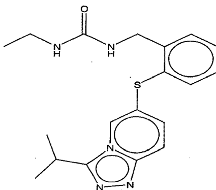
Y1X
