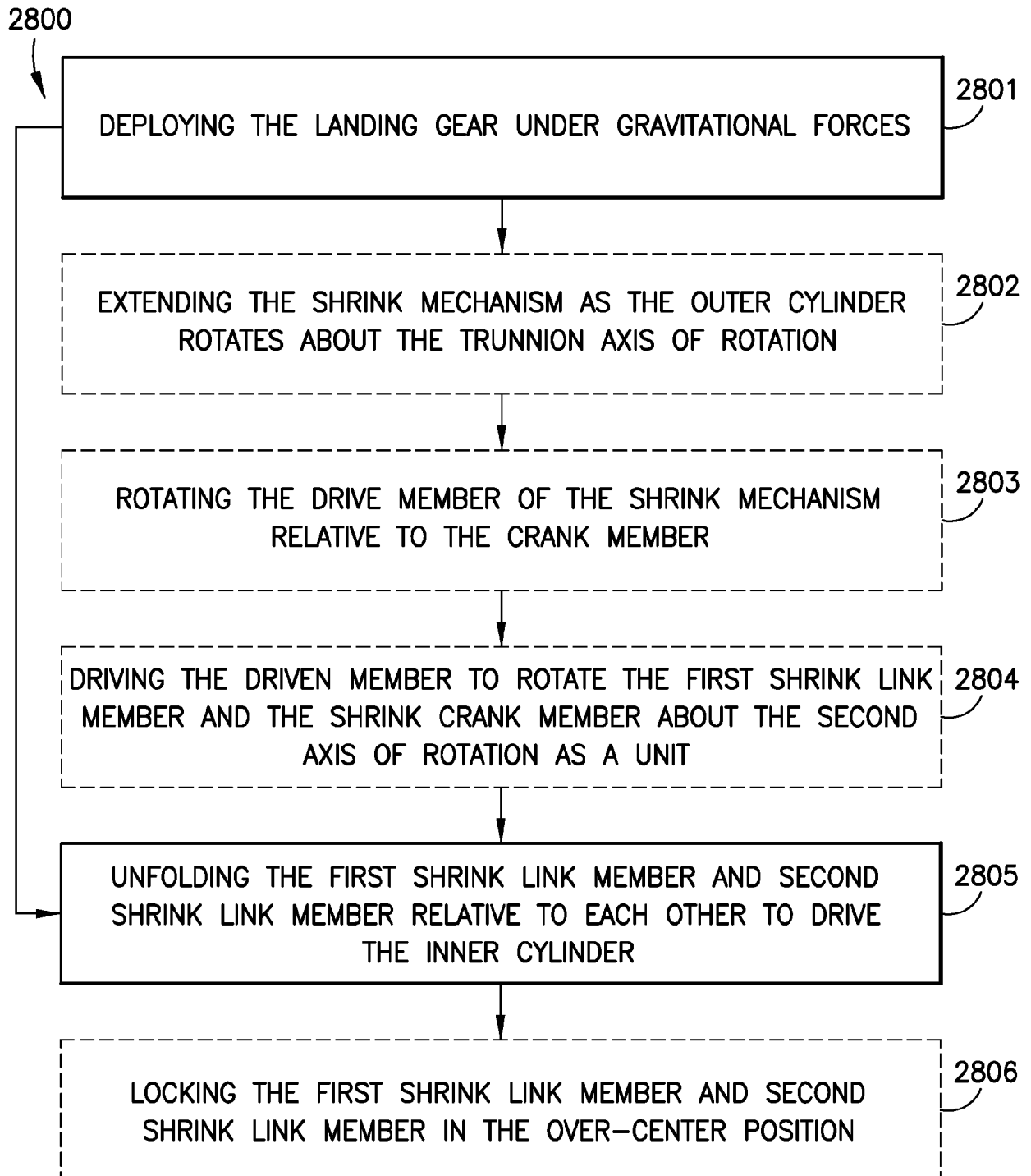
FIG.28
