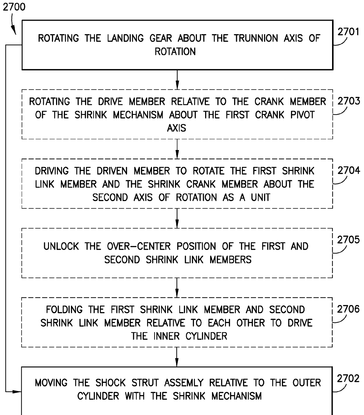
FIG.27
