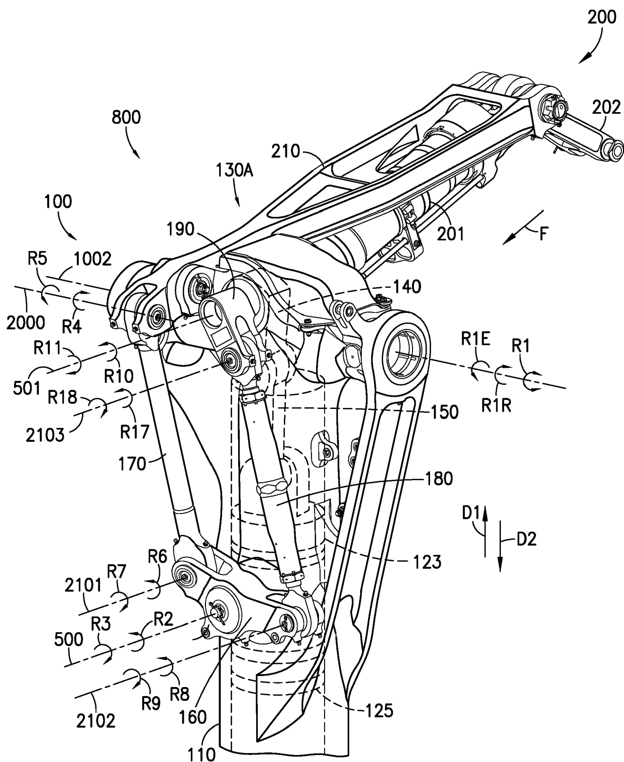
FIG.25A
