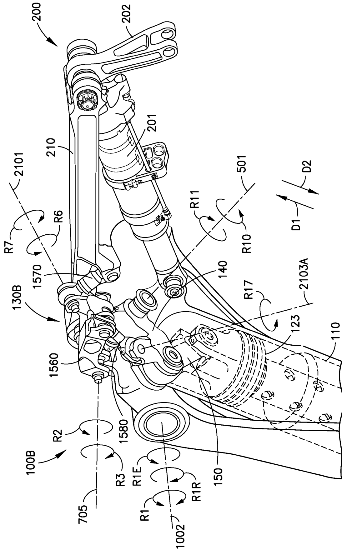
FIG. 26B
