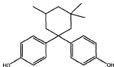
1,1-bis(4-hydroxyphenyl)-3,3,5-trimethyl-cyclohexane
