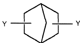
norbornane
