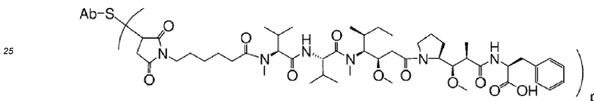
Ab-MC-MMAF
