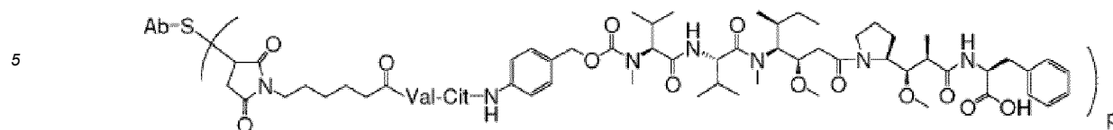
Ab-MC-vc-PAB-MMAF
