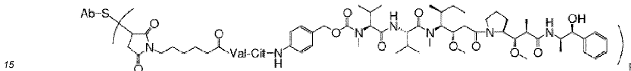
Ab-MC-vc-PAB-MMAE
