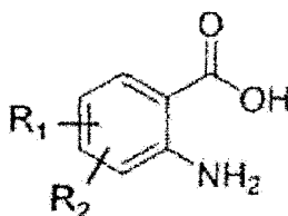
[Formule chimique 3]
