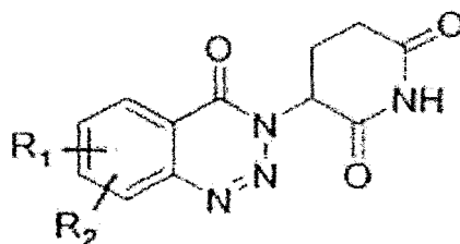
[Formule chimique 5]
