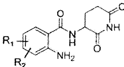
[Formule chimique 5]
