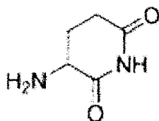
[Formule chimique 4]
