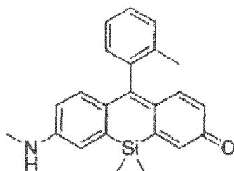
N-Me Si-Rhodol
