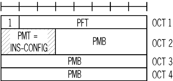
INS-CONFIG MESSAGE
