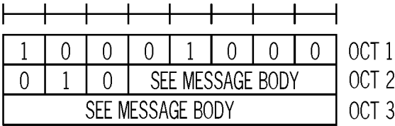
INS-CONFIG MESSAGE
