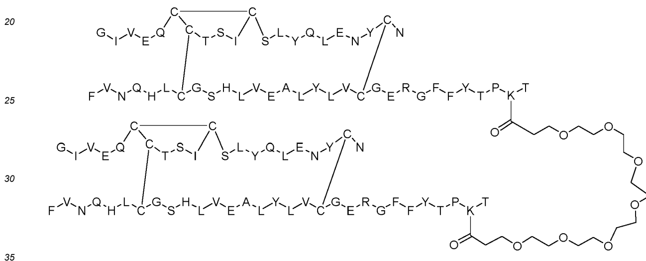
Dimer 15;
