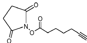
(Linker 8),
