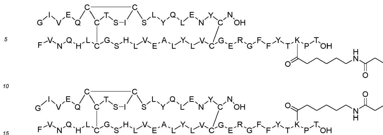
Dimer 35;
