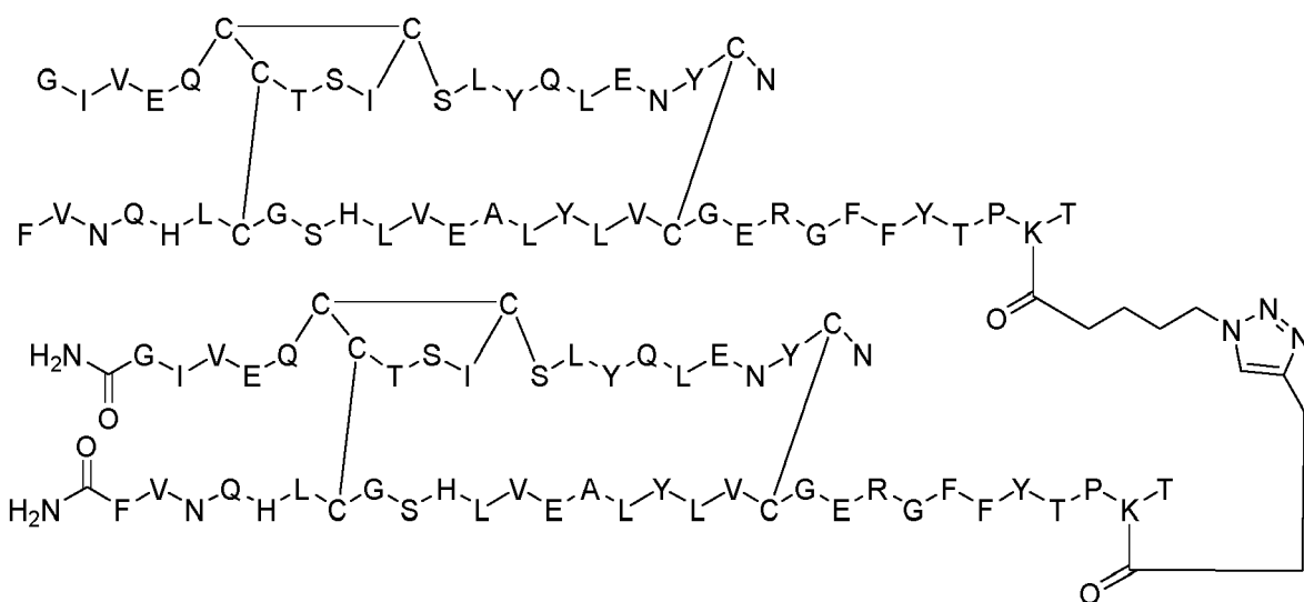
Dimer 46;
