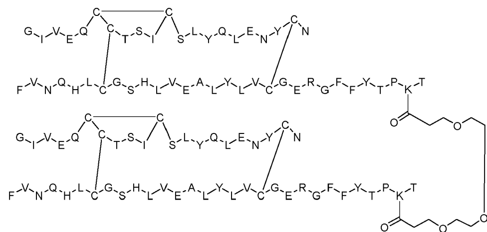
Dimer 5;
