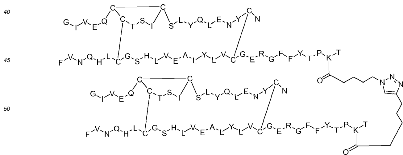
Dimer 57;
