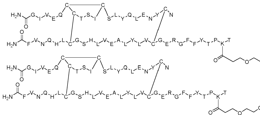
Dimer 10;
