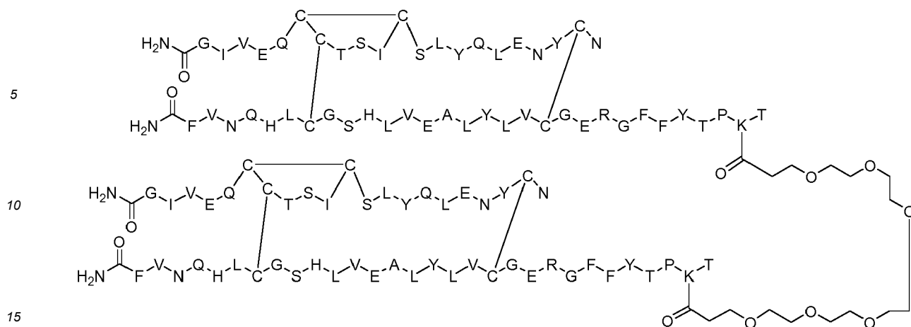
Dimer 14;
