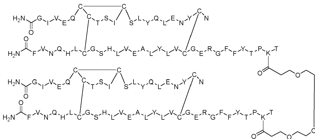
Dimer 10;
