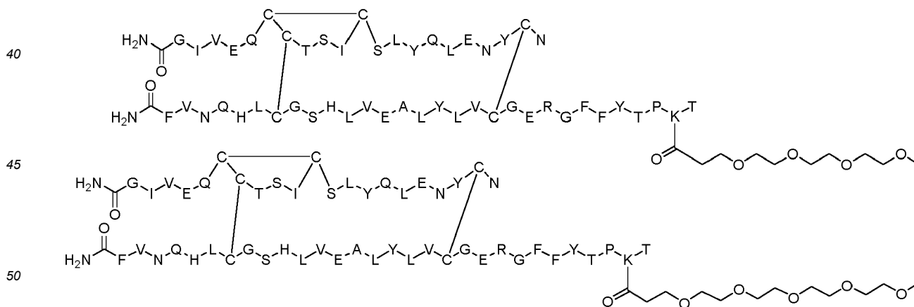
Dimer 16;
