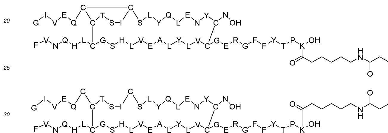
Dimer 30;
