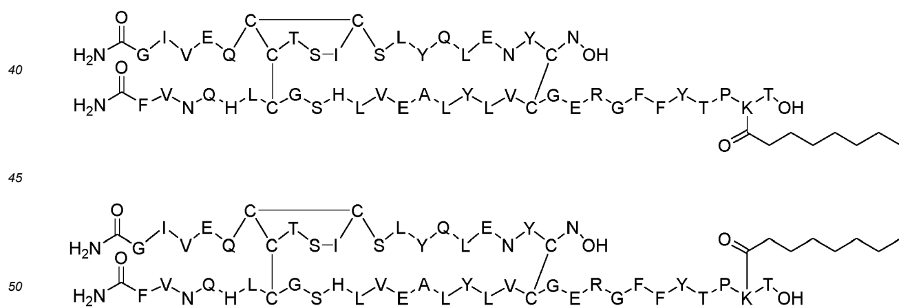
Dimer 37;
