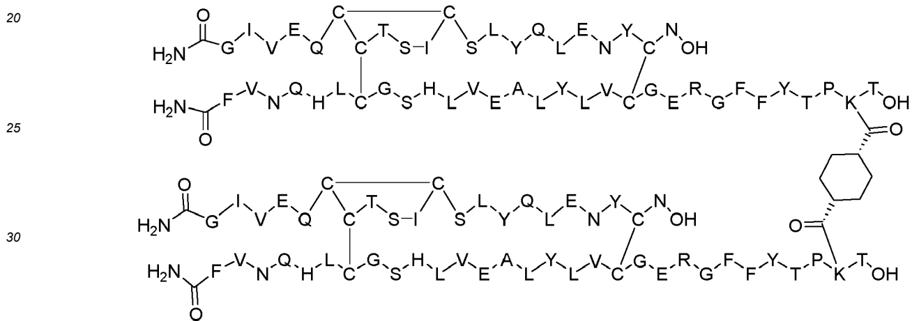
Dimer 78;
