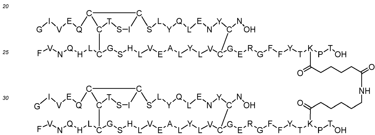
Dimer 33;
