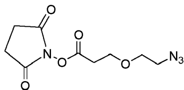
(Linker 7),
