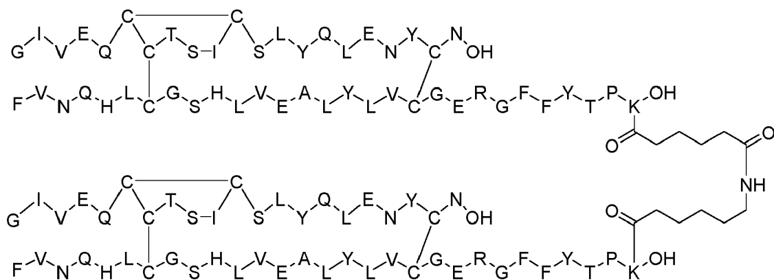
Dimer 29;
