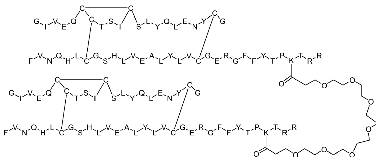
Dimer 53;
