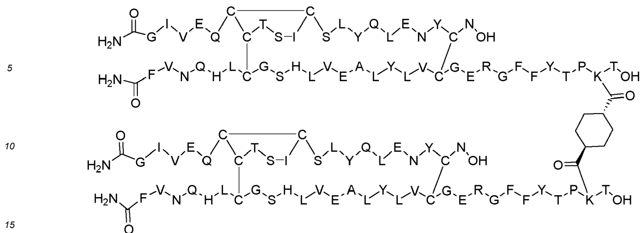
Dimer 77;
