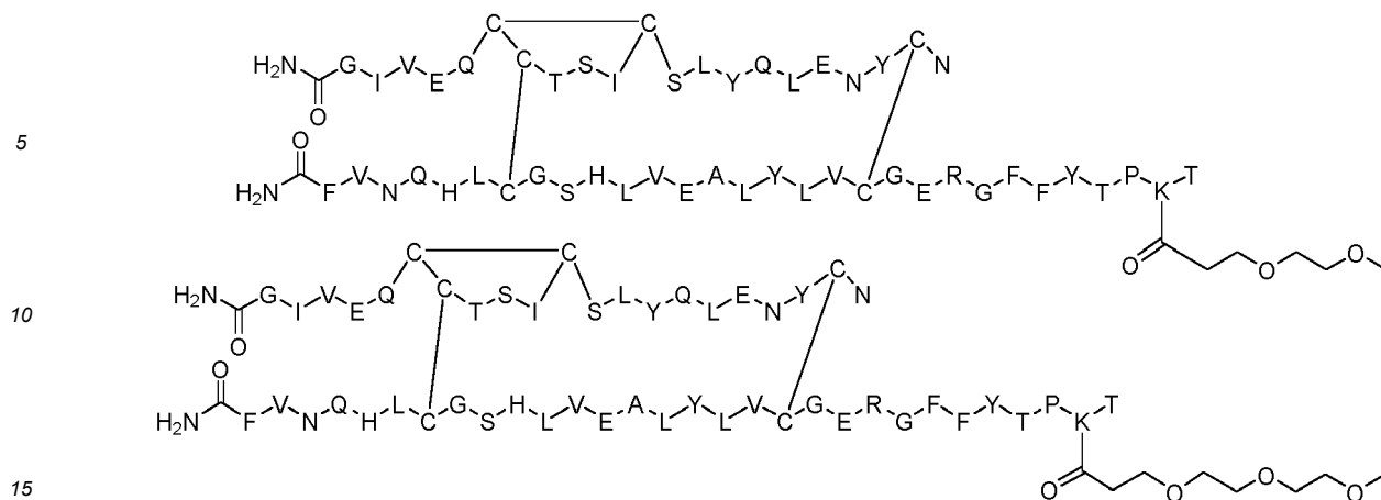
Dimer 11;
