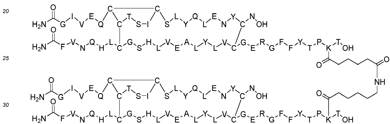
Dimer 21;
