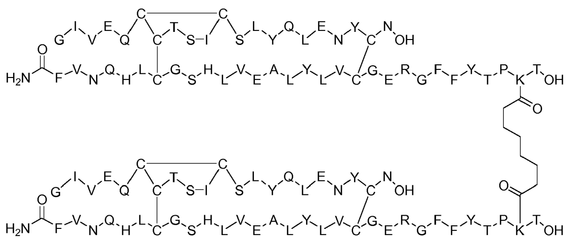
Dimer 54;
