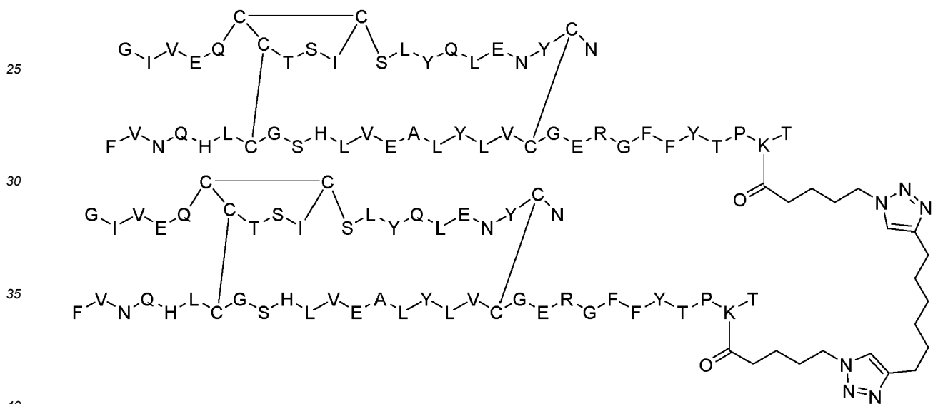
Dimer 42;
