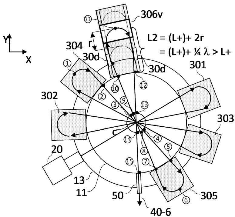
FIG.3(d2) 6 MeV
