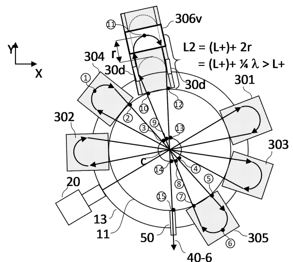
FIG.3(d2) 6 MeV
