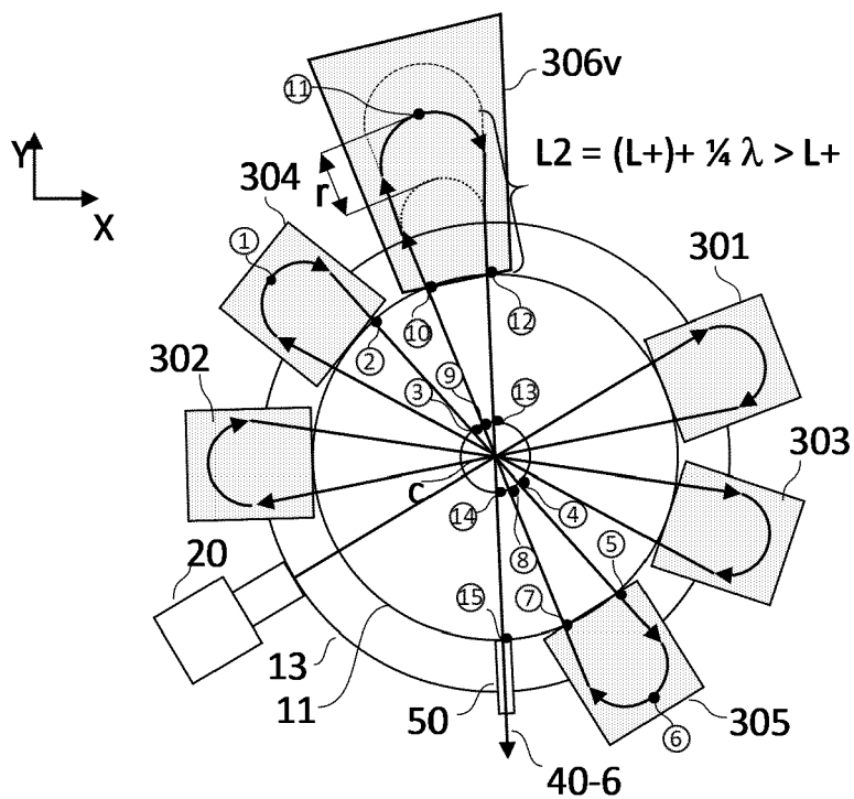
FIG.3(d3) 6 MeV
