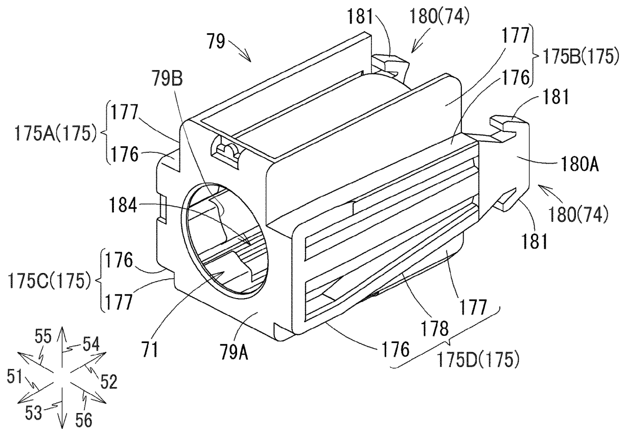
[Fig. 13B]
