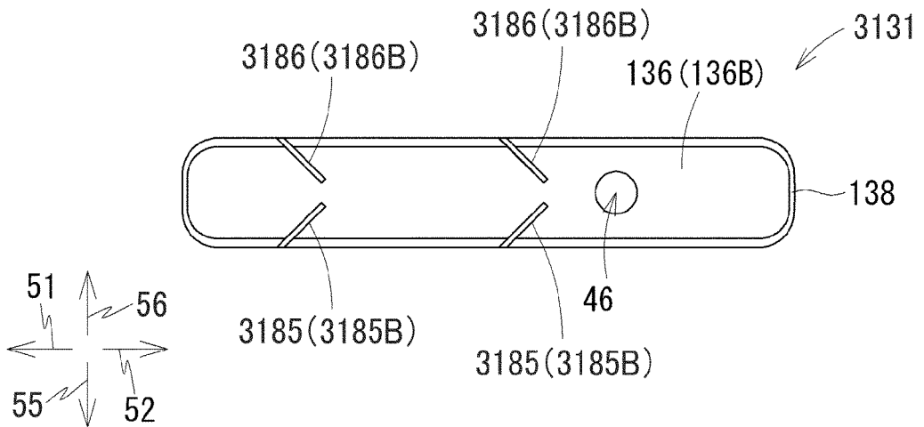
[Fig. 26C]
