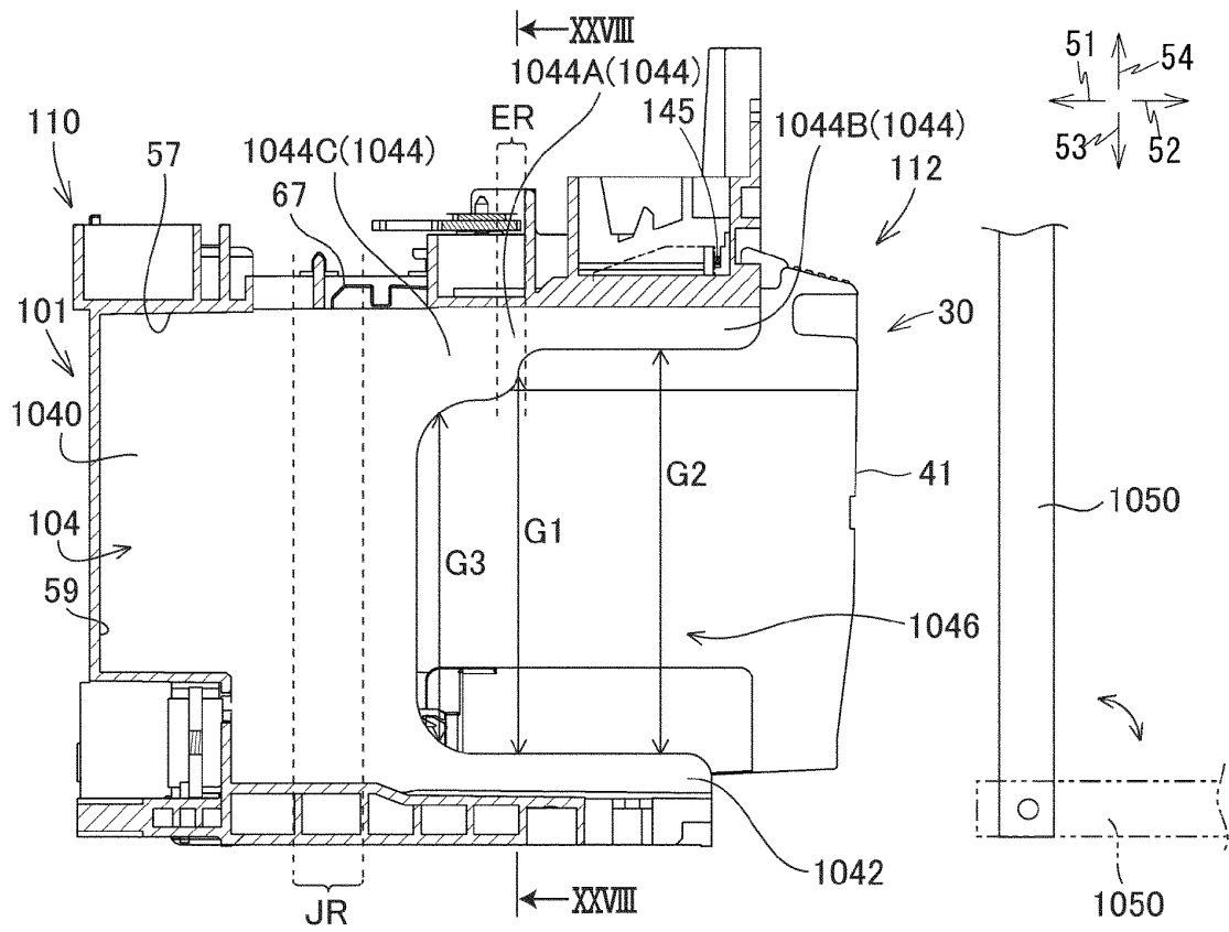
[Fig. 27B]
