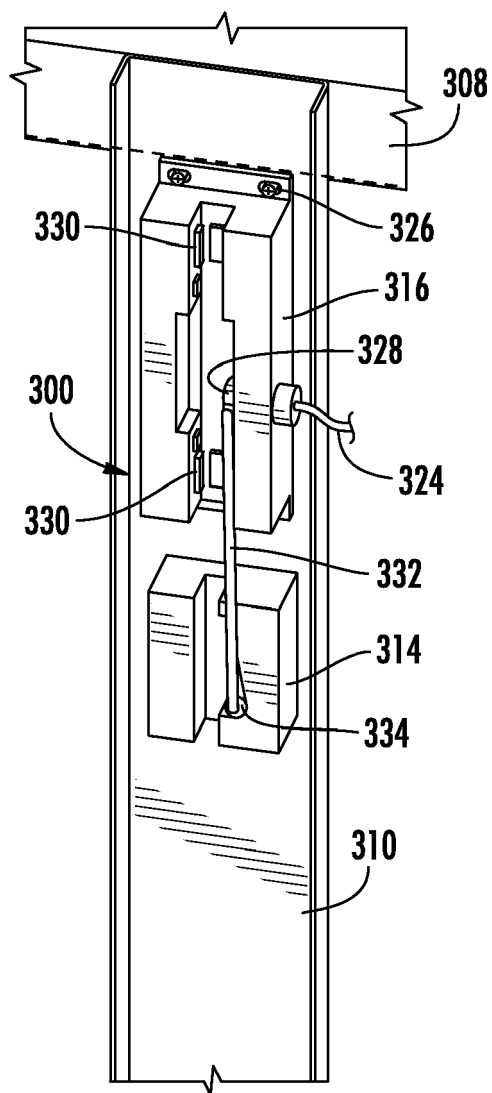
FIG. 3C
