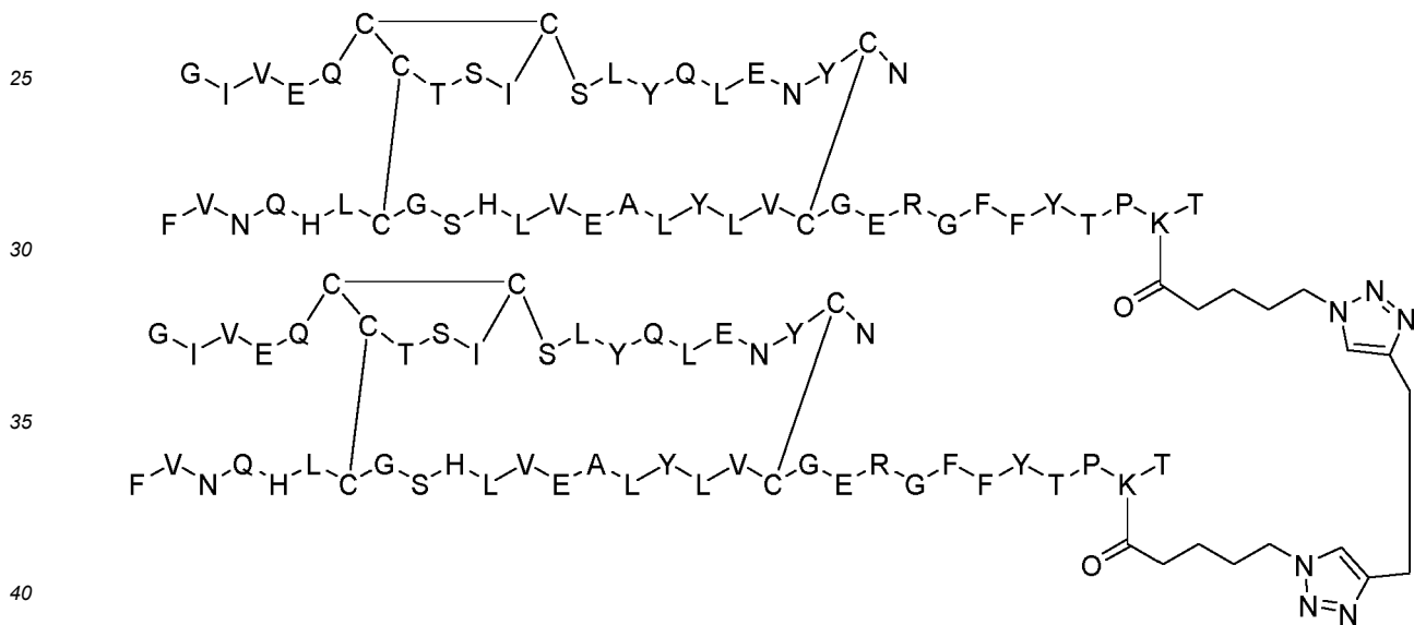
Dimer 44;
