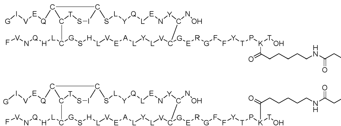
Dimer 25;
