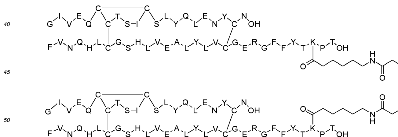
Dimer 35;
