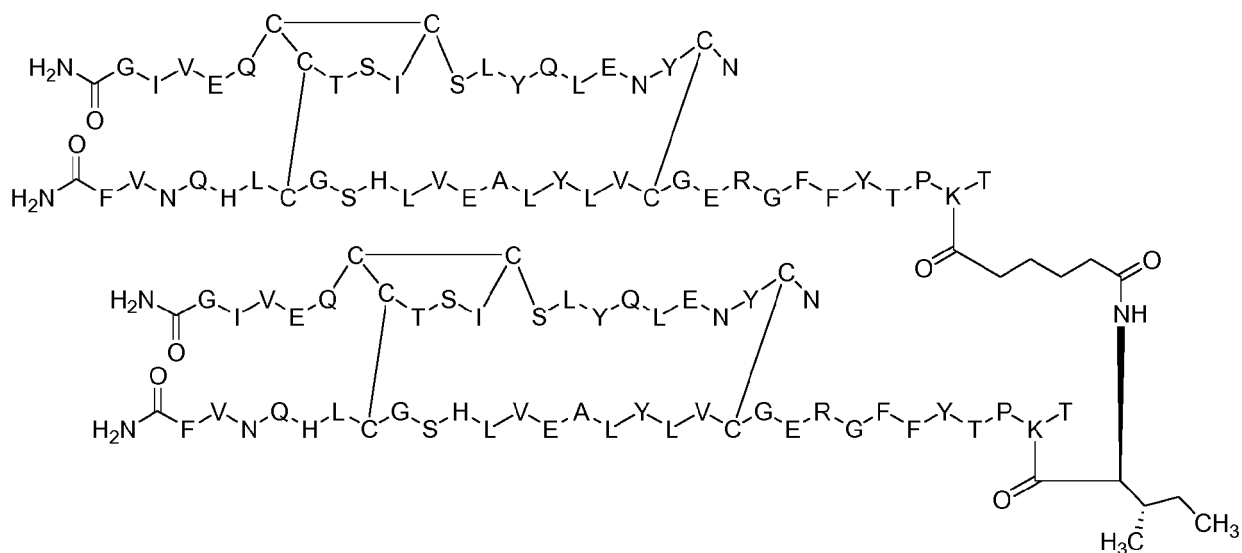
Dimer 63;
