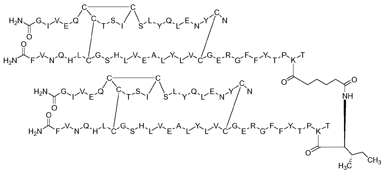
Dimer 63;
