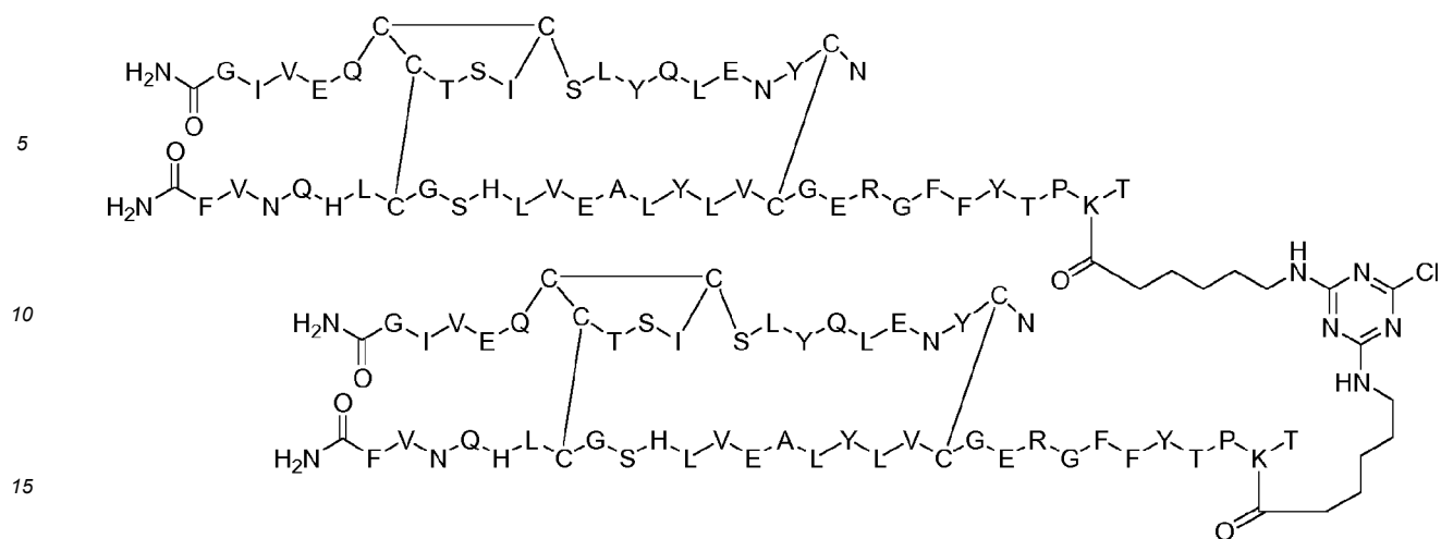
Dimer 74;
