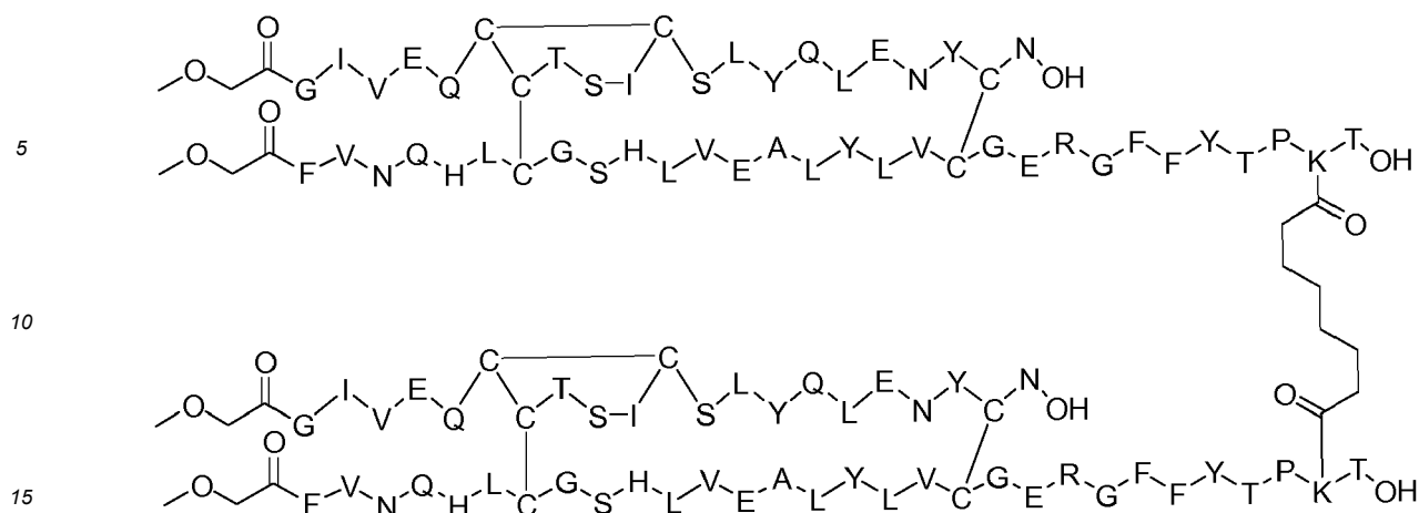
Dimer 56;
