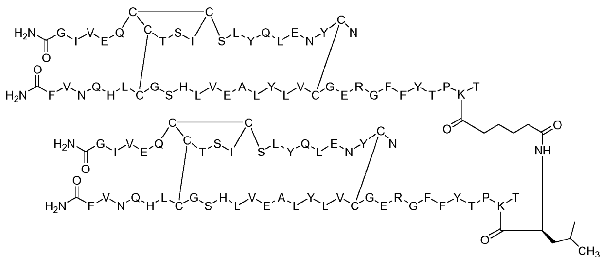
Dimer 64;
