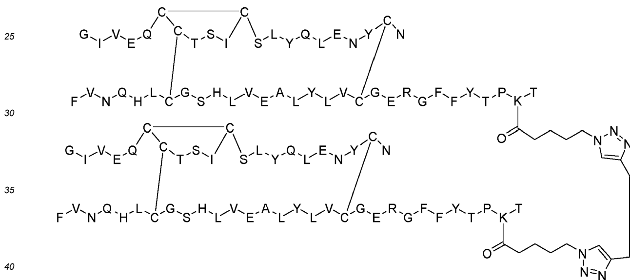
Dimer 44;
