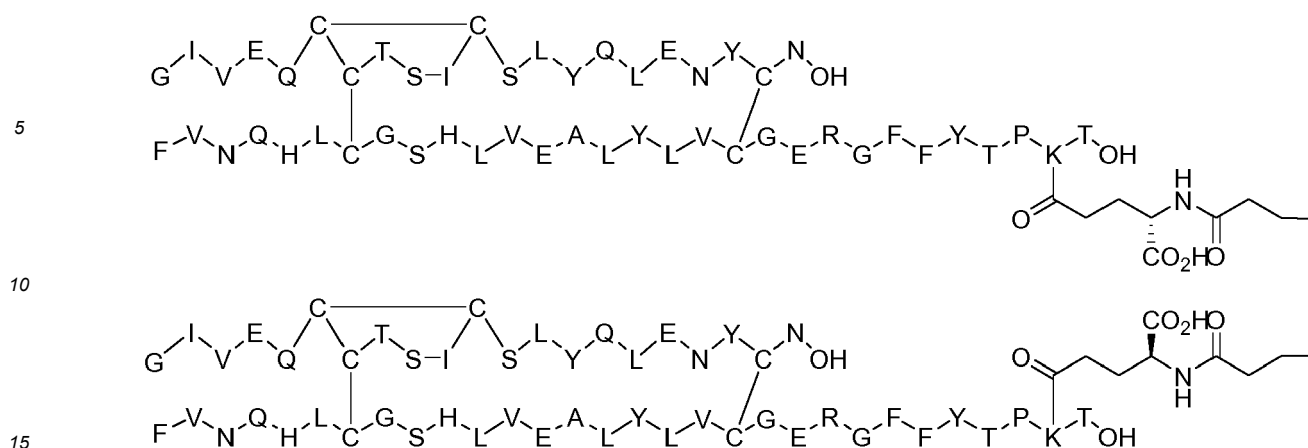
Dimer 36;
