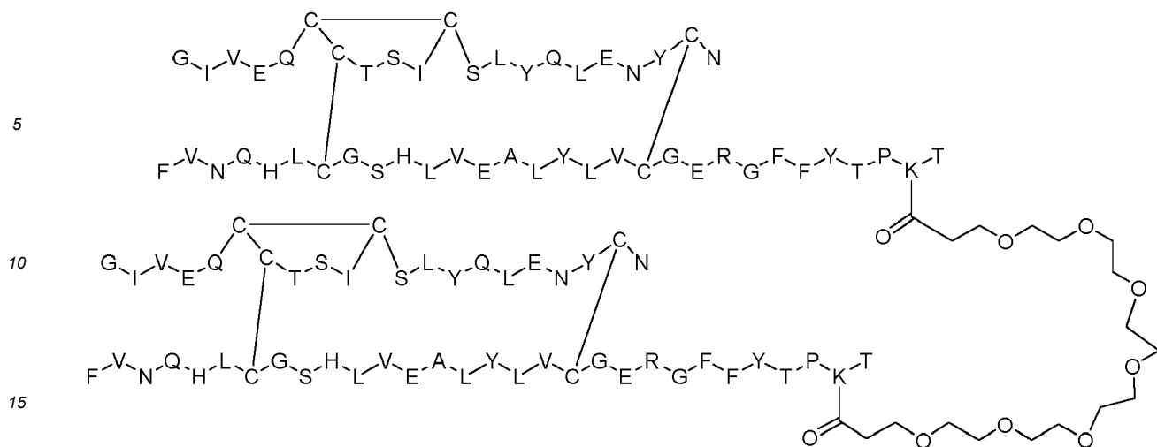
Dimer 15;
