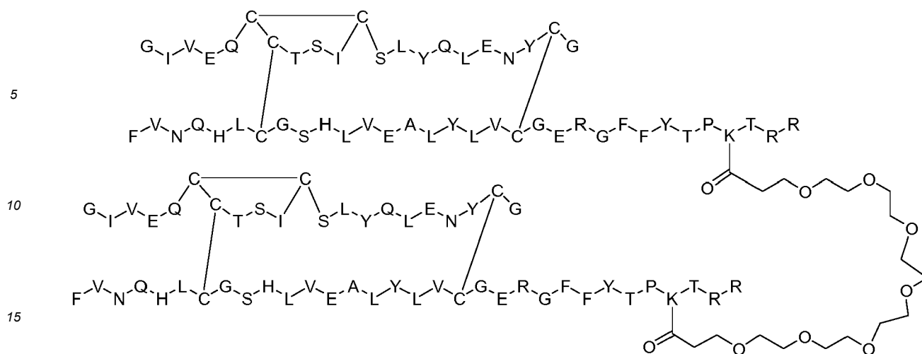
Dimer 53;
