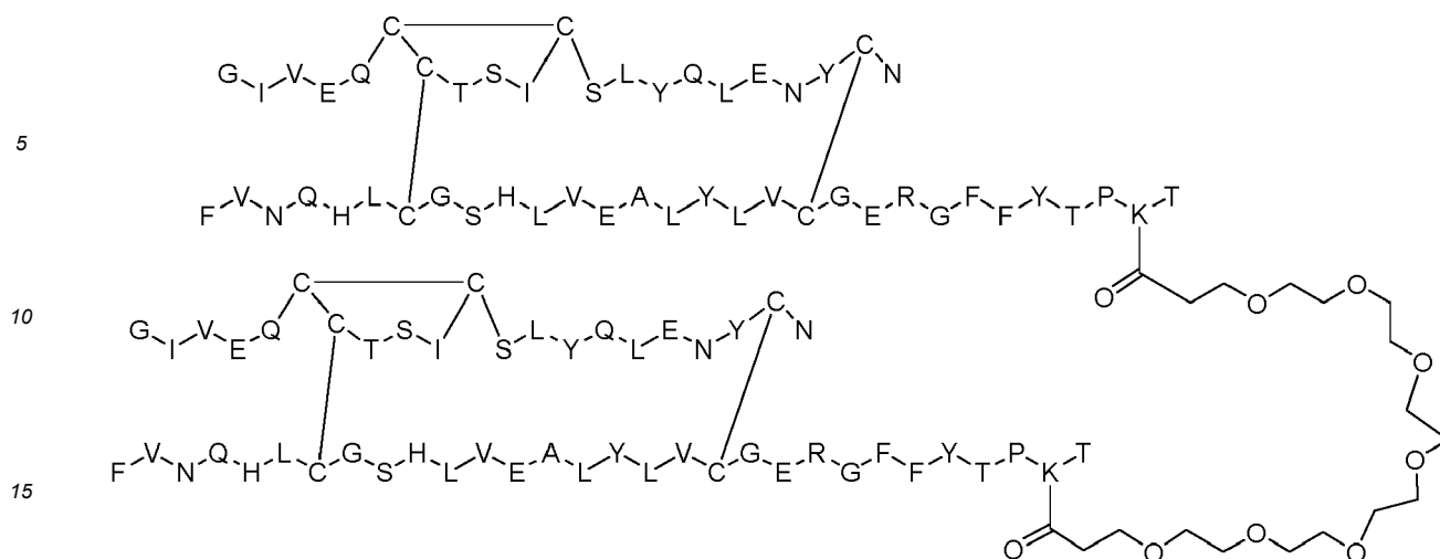
Dimer 15;
