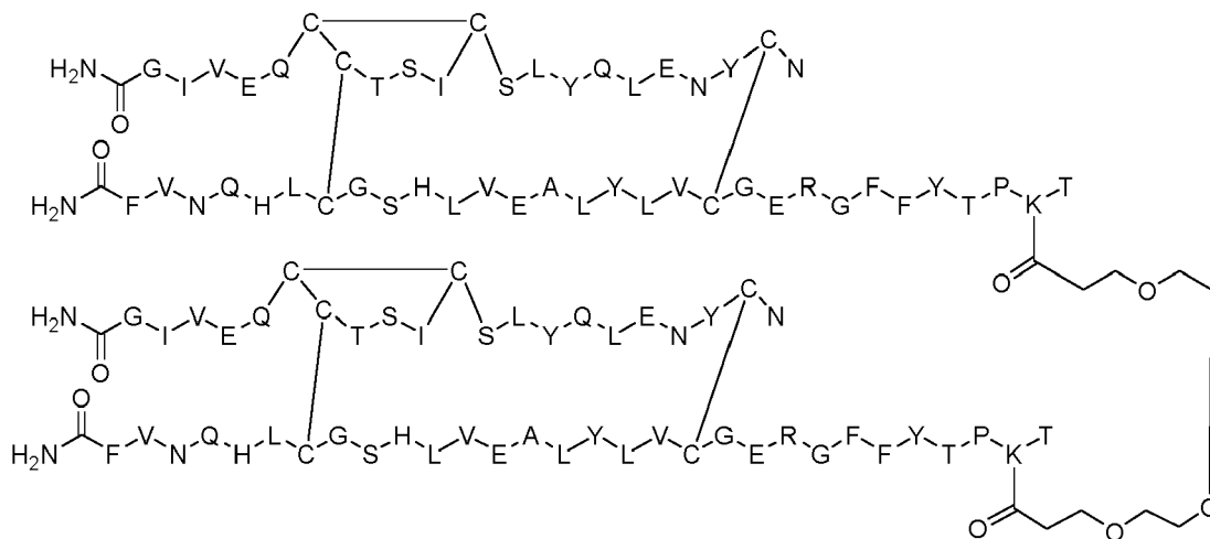
Dimer 10;
