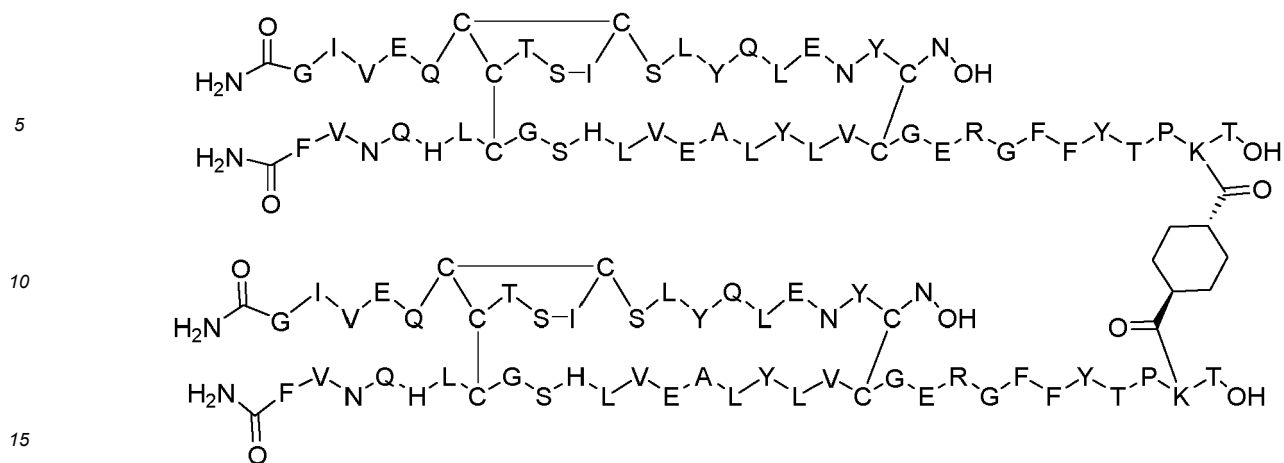
Dimer 77;
