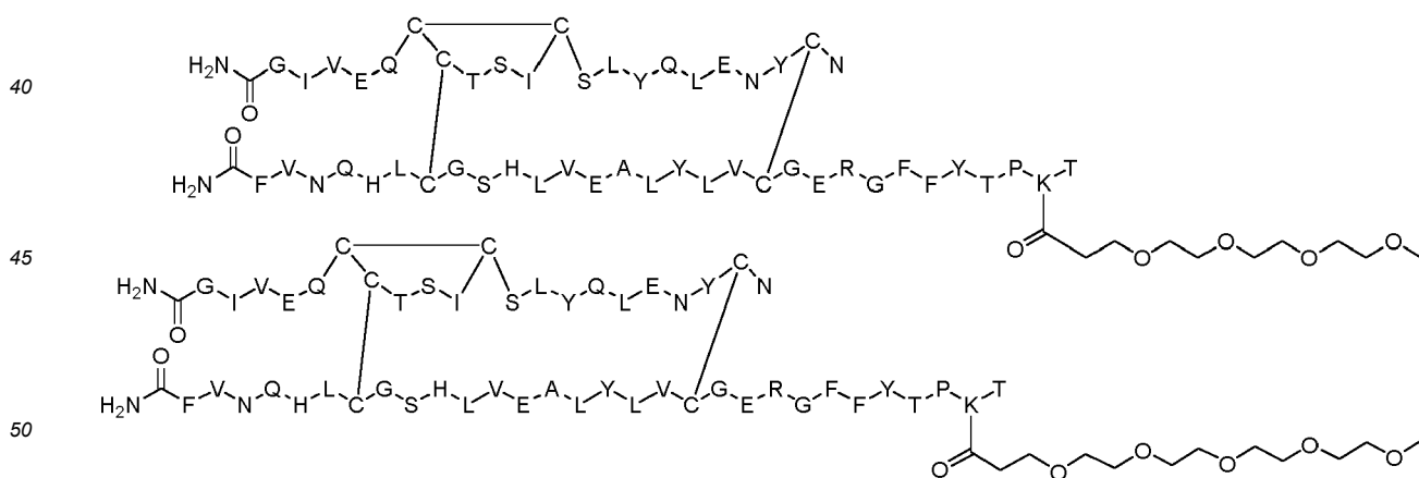
Dimer 15;
