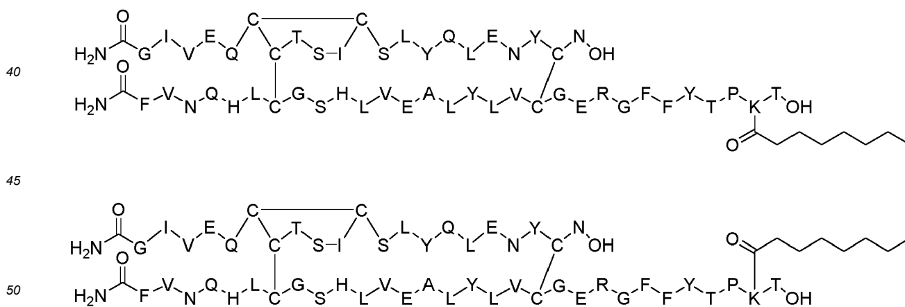
Dimer 37;
