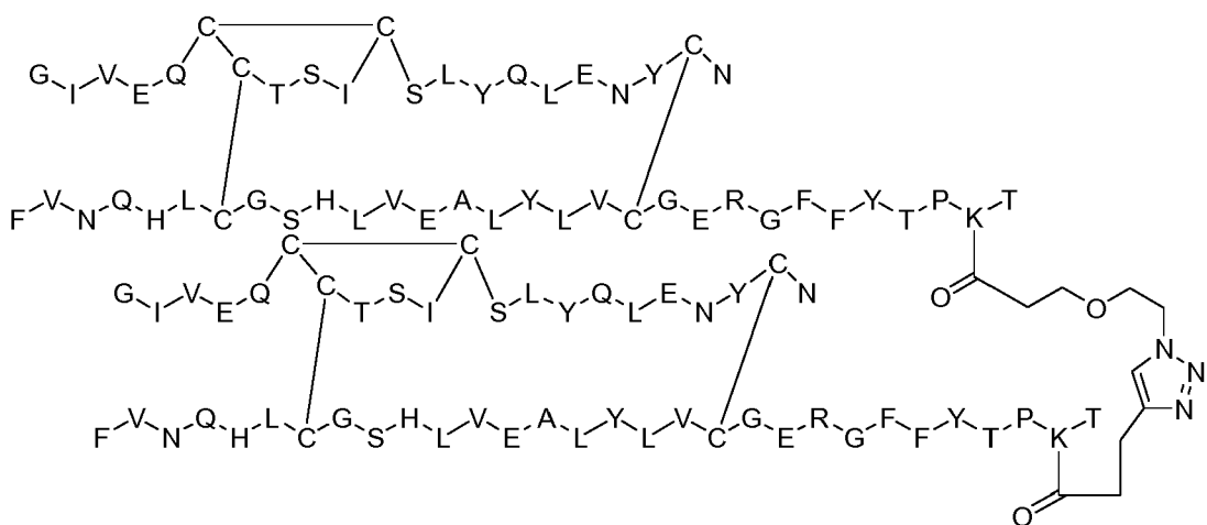
Dimer 80;
