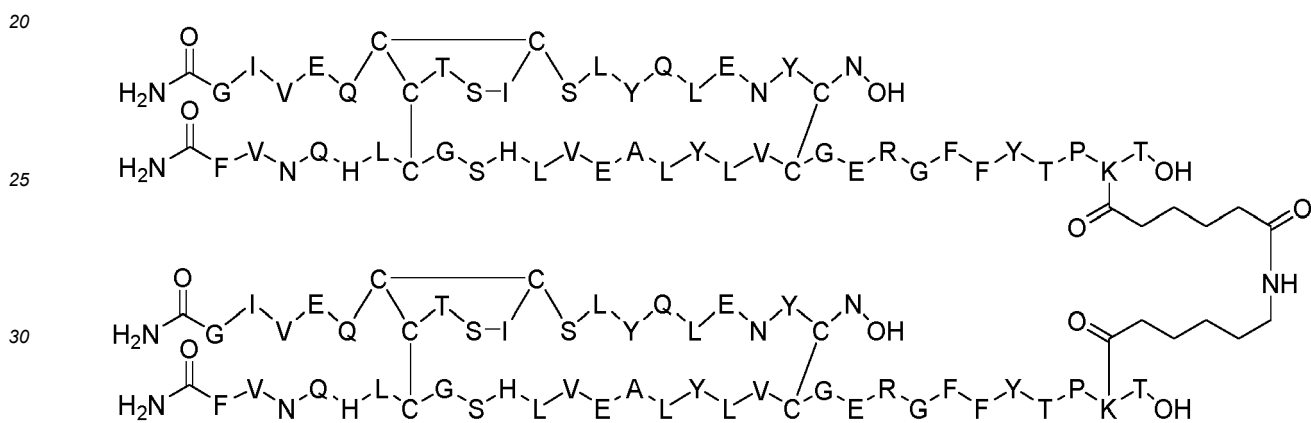
Dimer 21;
