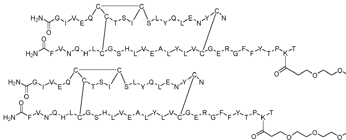
Dimer 11;
