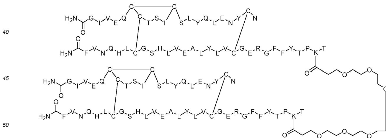
Dimer 14;
