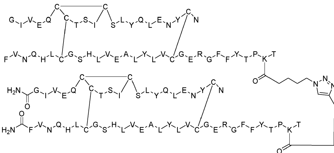
Dimer 46;
