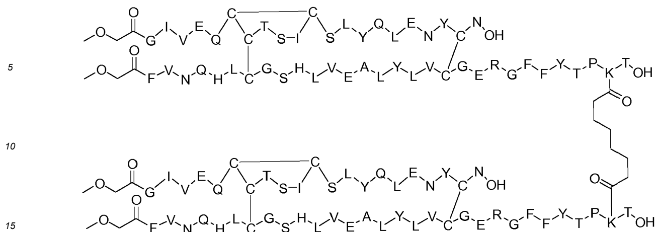
Dimer 56;
