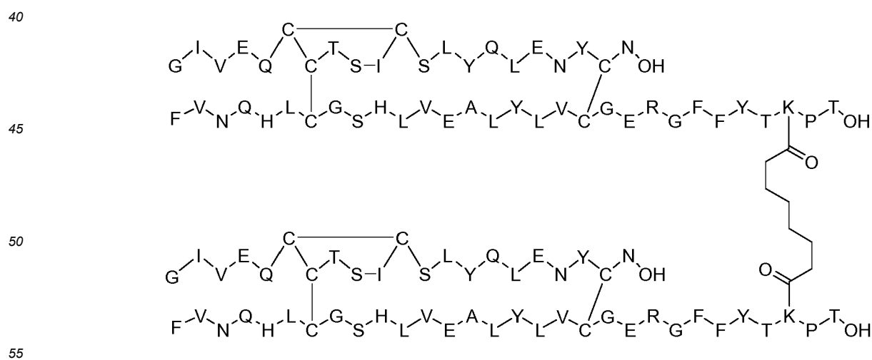
Dimer 16;
