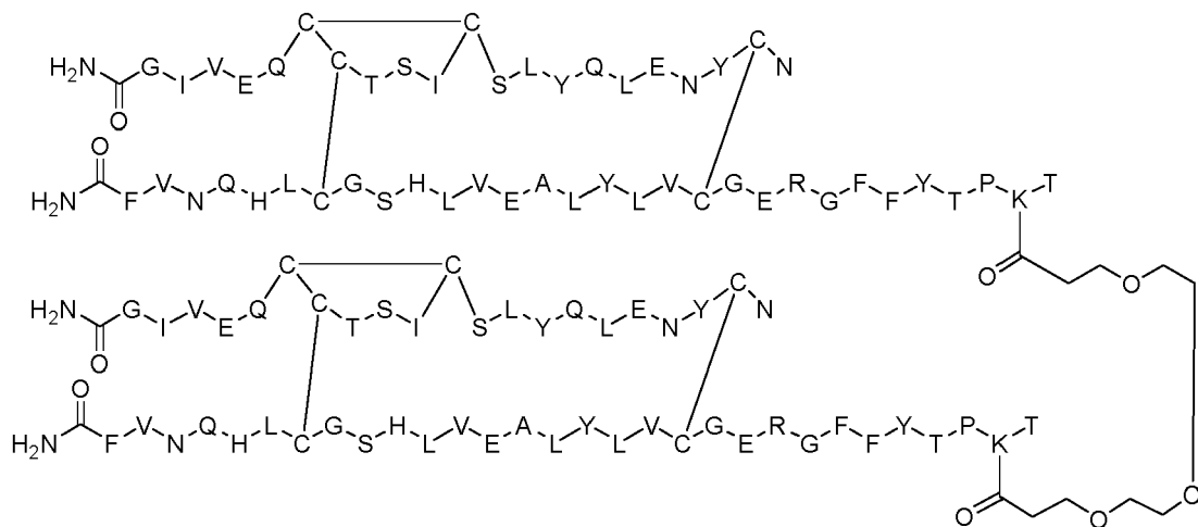
Dimer 10;
