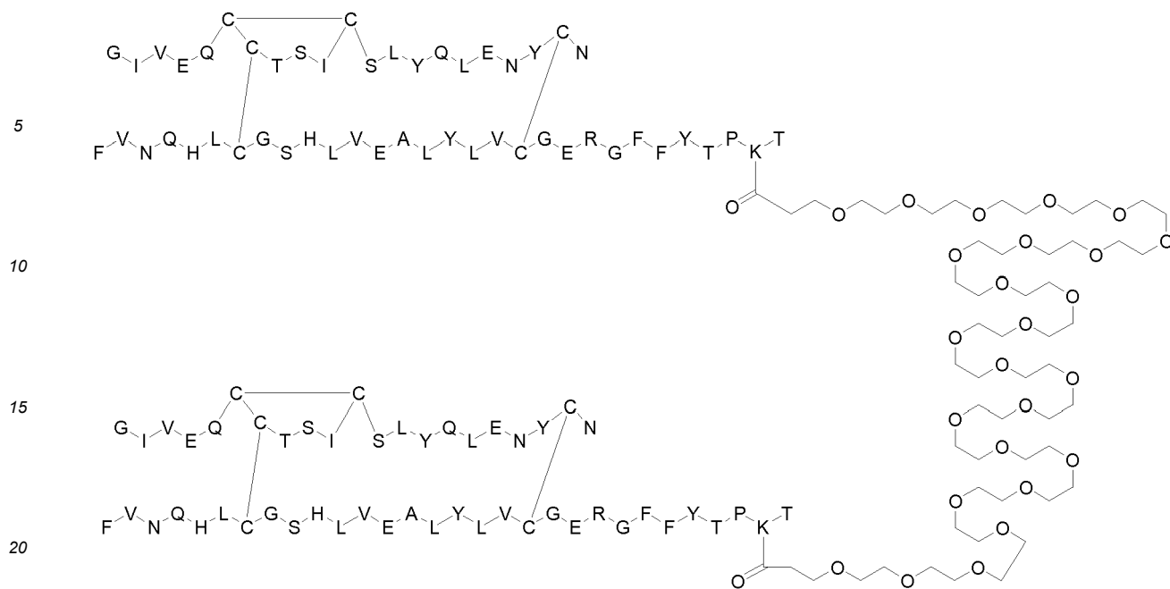
Dimer 85;
