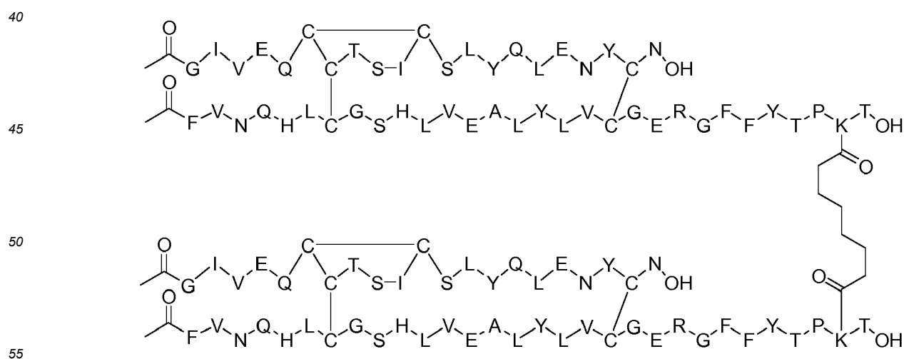
Dimer 55;
