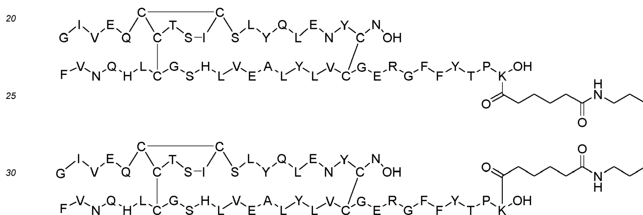
Dimer 31;
