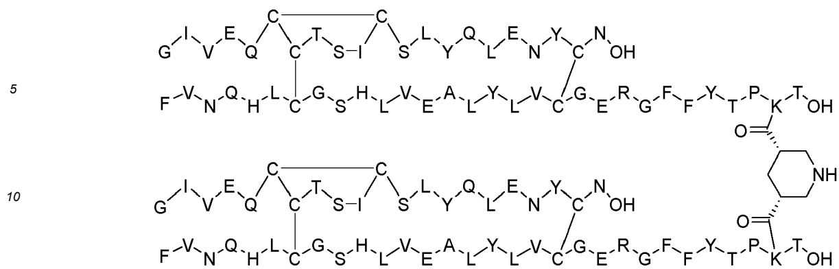
Dimer 81;
