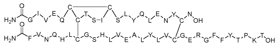
Dimer 2;
