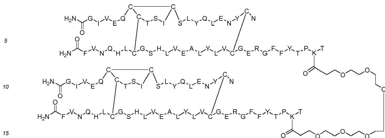
Dimer 14;
