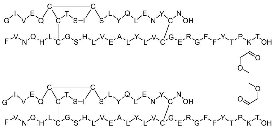
Dimer 1;
