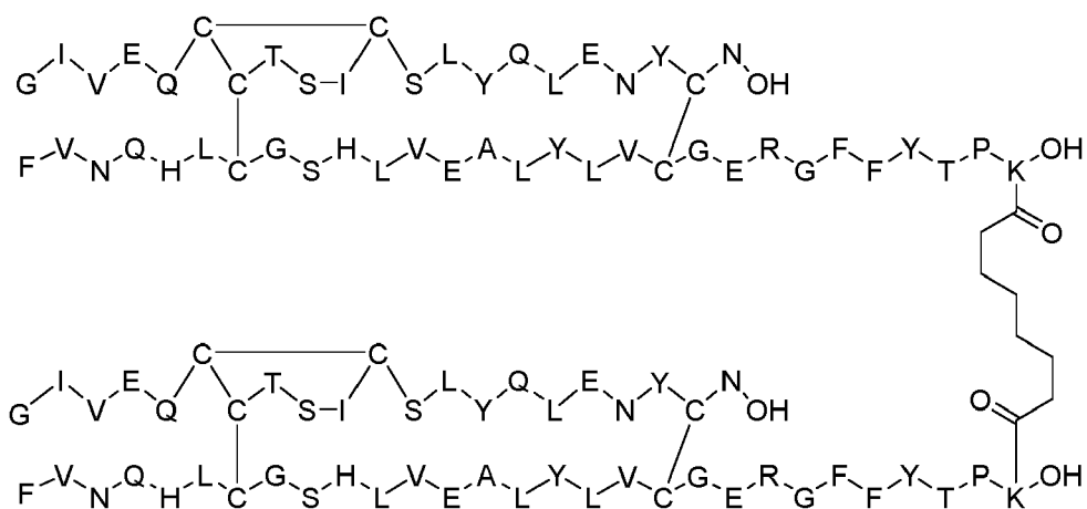
Dimer 20;
