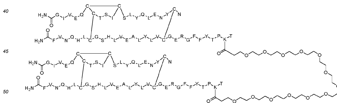
Dimer 17;
