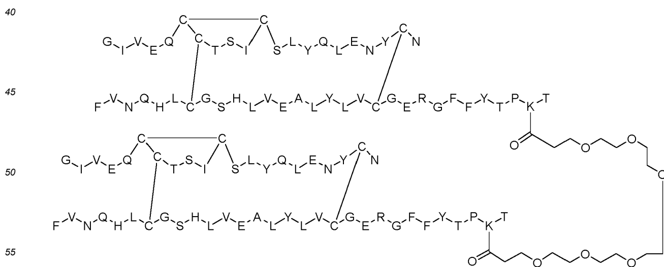
Dimer 76;
