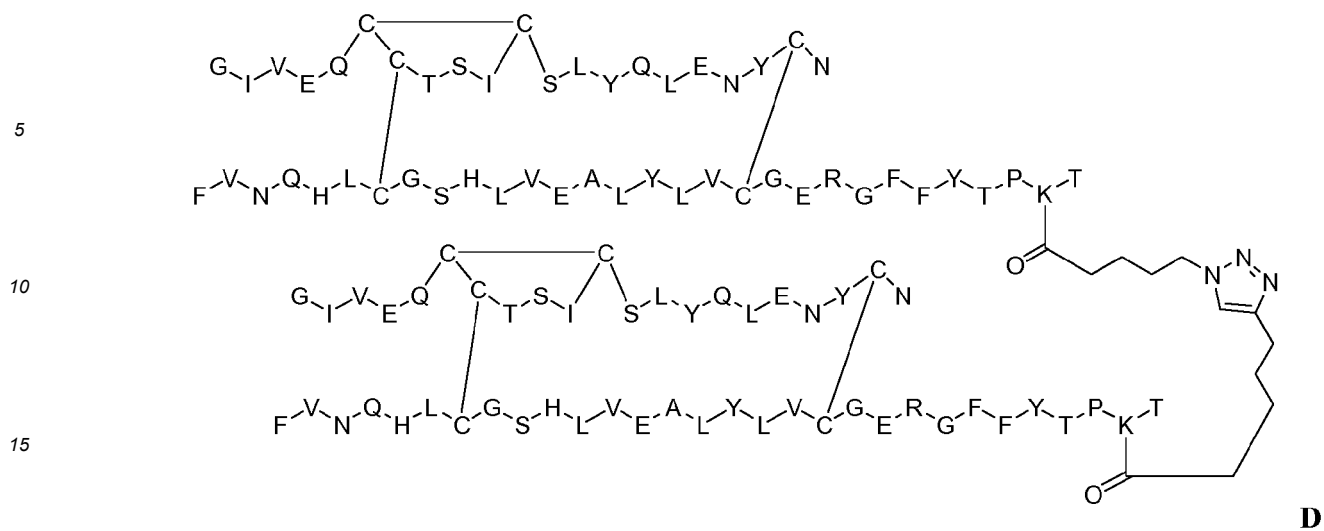
Dimer 57;
