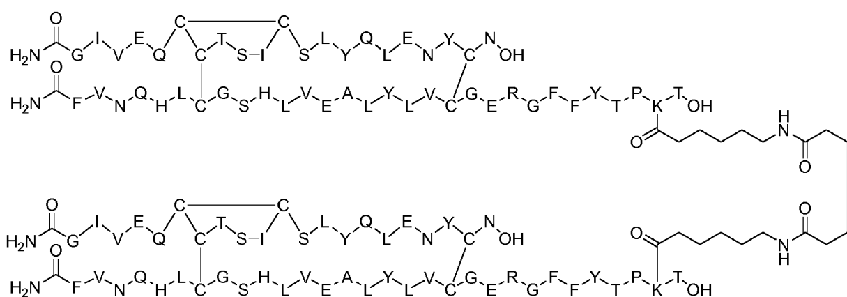
Dimer 23;
