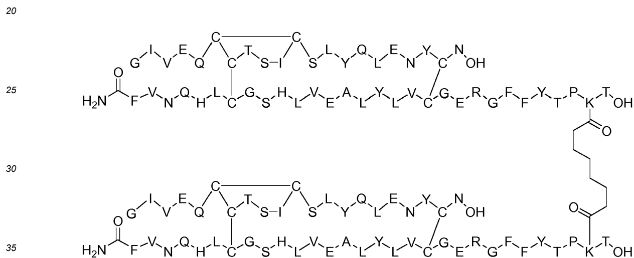
Dimer 54;
