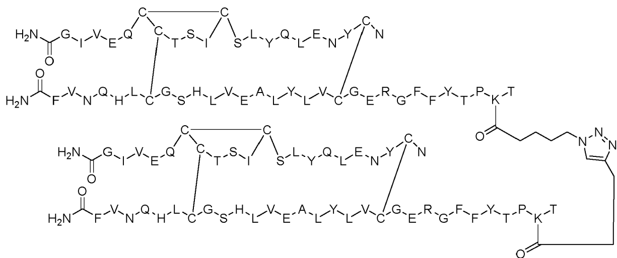
Dimer 47;
