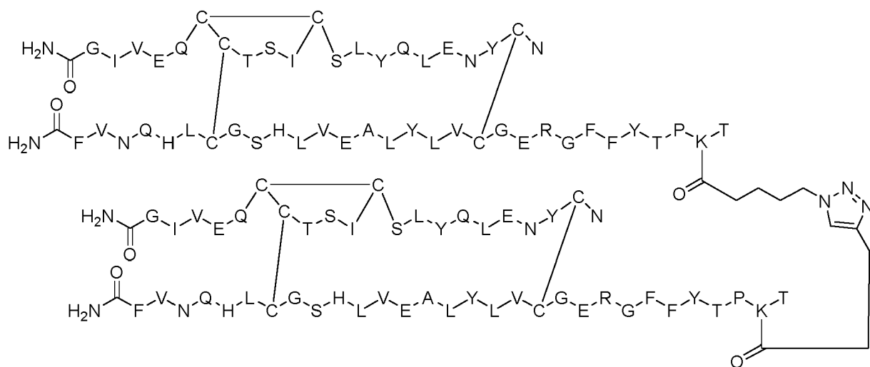
Dimer 47;
