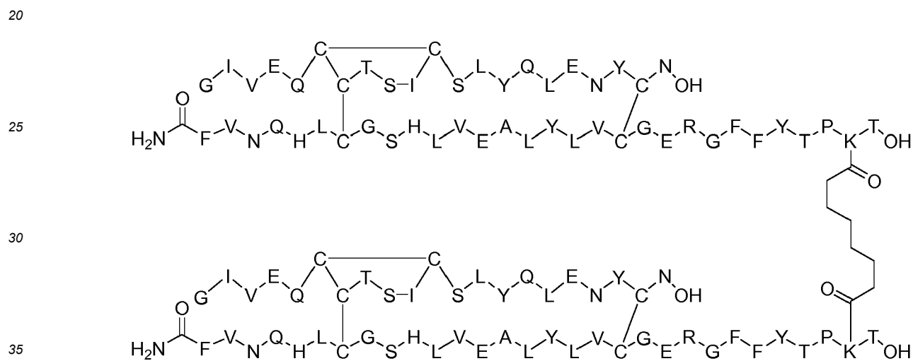
Dimer 54;
