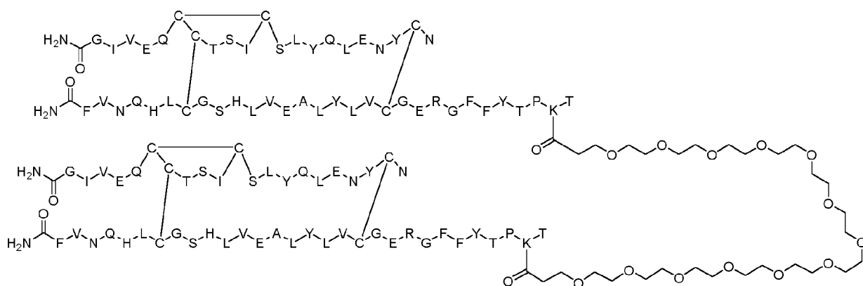
Dimer 17;
