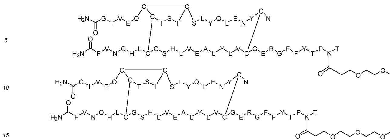
Dimer 11;
