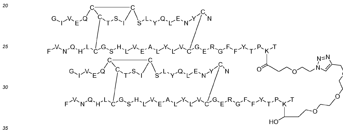
Dimer 79;
