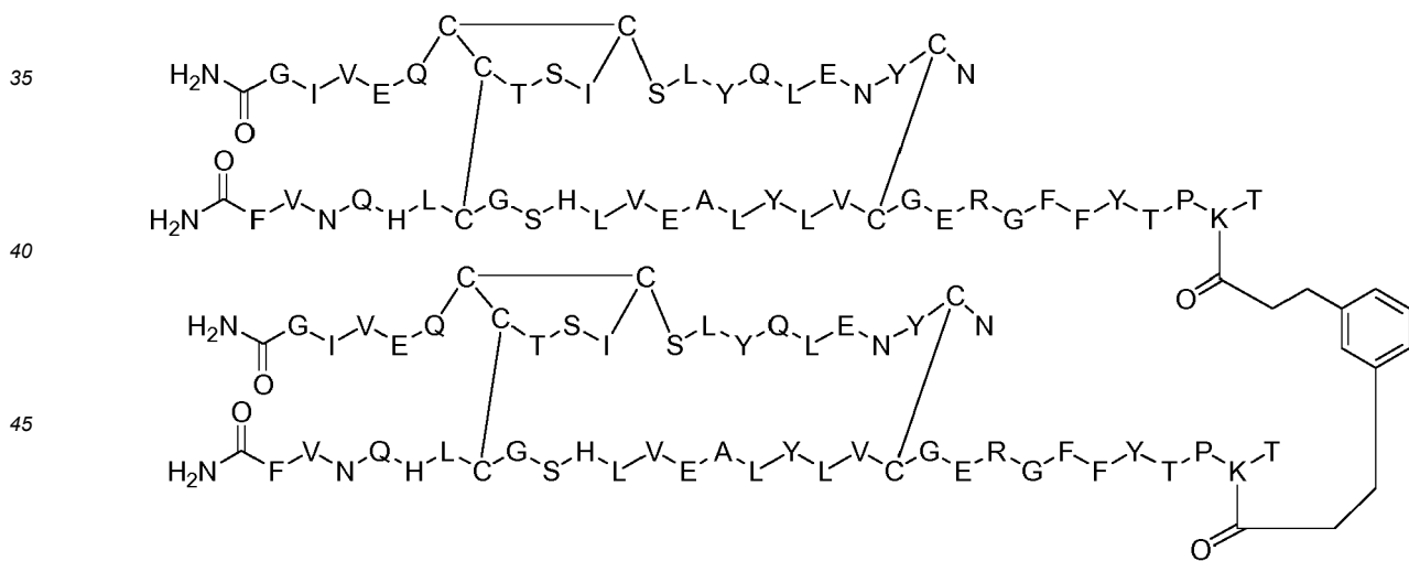
Dimer 73;
