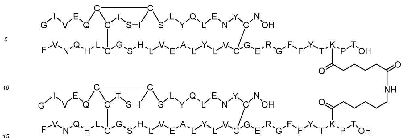
Dimer 33;
