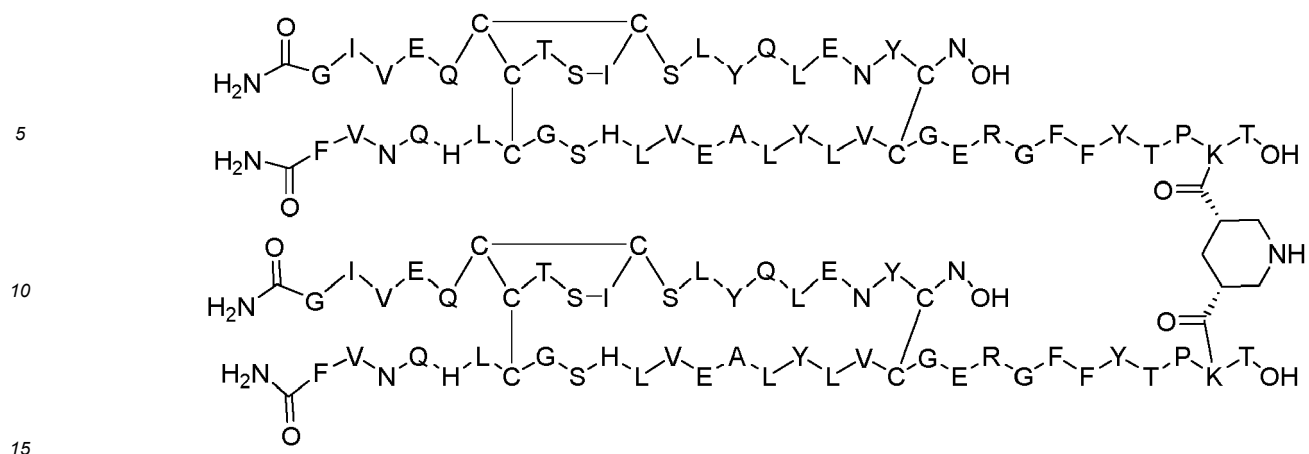
Dimer 86;
