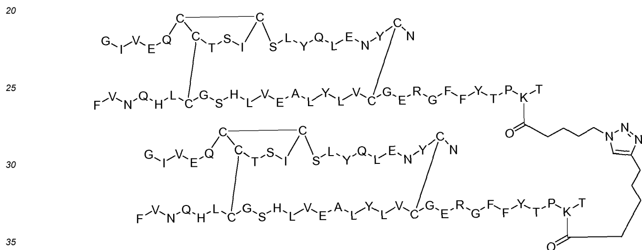
Dimer 57;
