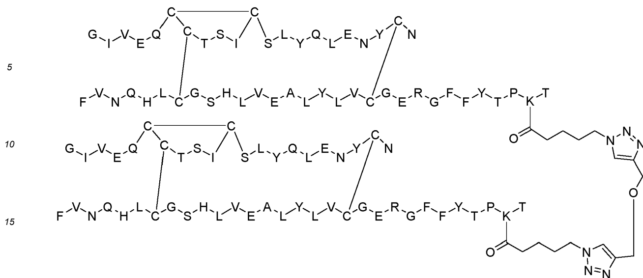
Dimer 43;
