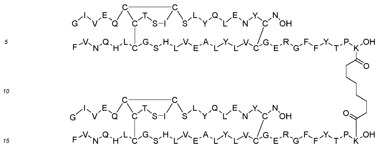
Dimer 20;
