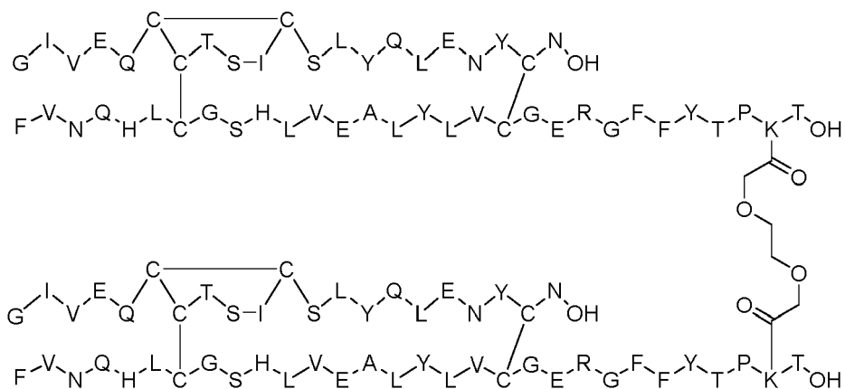
Dimer 1;
