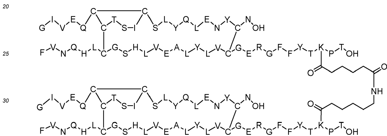
Dimer 33;
