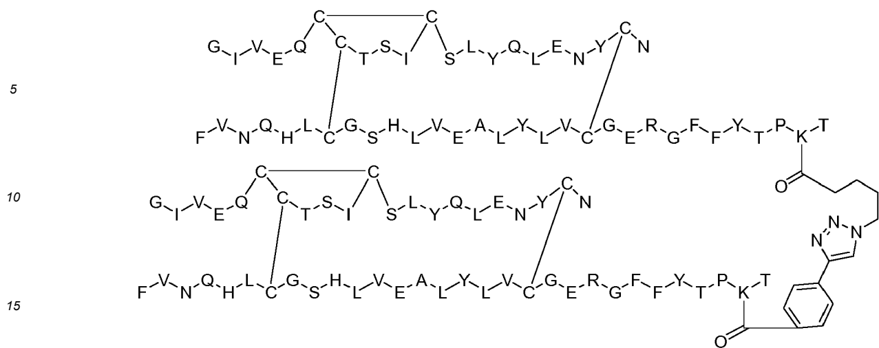
Dimer 75;
