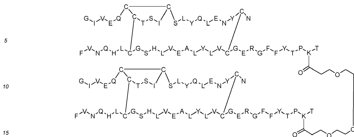
Dimer 5;
