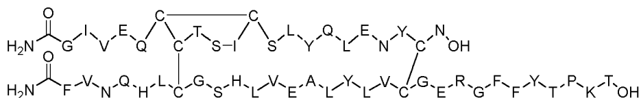
Dimer 2;
