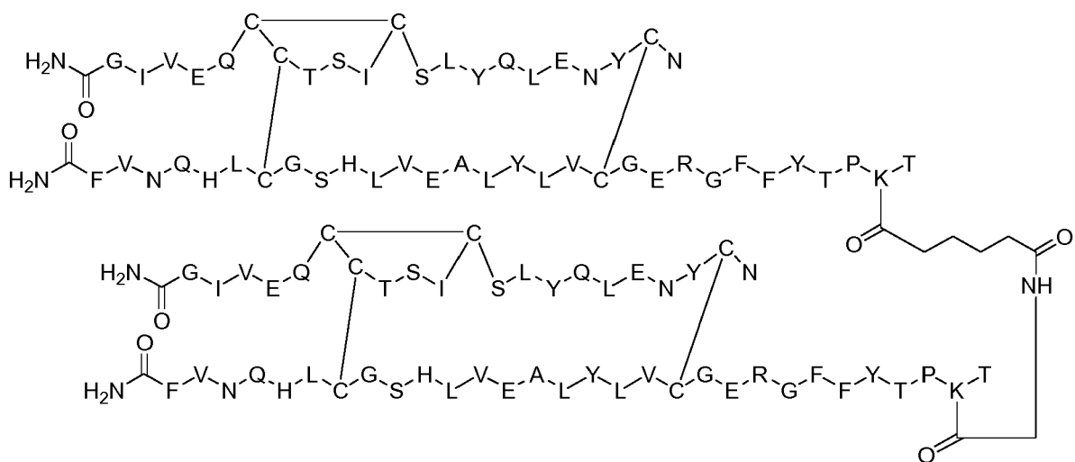
Dimer 61;
