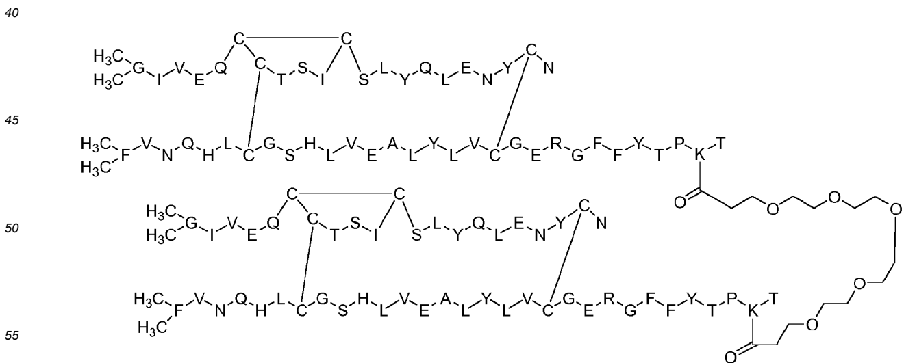
Dimer 67;
