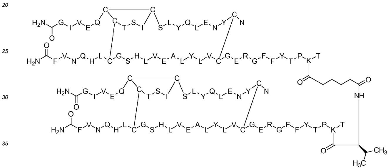
Dimer 66;
