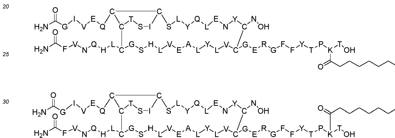
Dimer 37;
