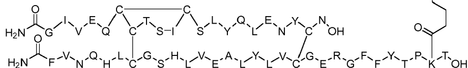
Dimer 2;
