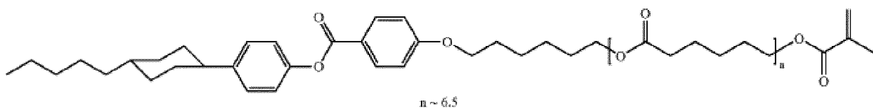
1-(6-(6-(6-(6-(6-(6-(4-(4-(trans-4-pentylcyclohexyl)phenoxy)carbonyl)phenoxy)hexyloxy)-6-oxohexyloxy)-6-oxohexyloxy)-6-oxohexyloxy)-6-oxohexyloxy)-6-oxohexyloxy)-2-methylprop-2-en-1-one
