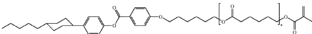
1-(6-(6-(6-(6-(6-(6-(6-(4-(4-(trans-4-pentylcyclohexyl)phenoxy)carbonyl)phenoxy)hexyloxy)-6-oxohexyloxy)-6-oxohexyloxy)-6-oxohexyloxy)-6-oxohexyloxy)-6-oxohexyloxy)-6-oxohexyloxy)-2-methylprop-2-en-1-one
