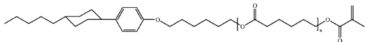
1-(6-(6-(6-(6-(4-(4-(trans-4-pentylcyclohexyl)phenoxy)hexyloxy)-6-oxohexyloxy)-6-oxohexyloxy)-6-oxohexyloxy)-2-methylprop-2-en-1-one
