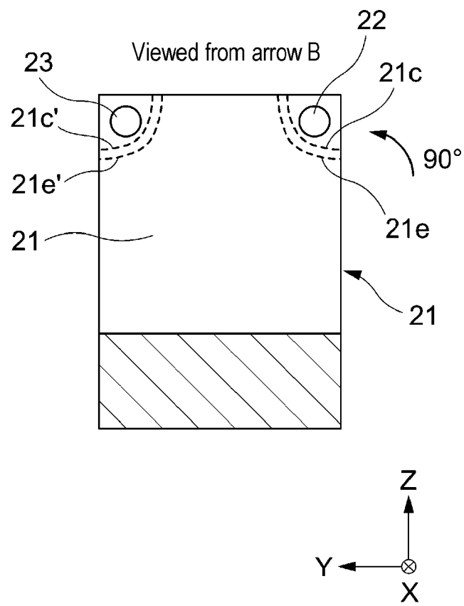
FIG. 9B
