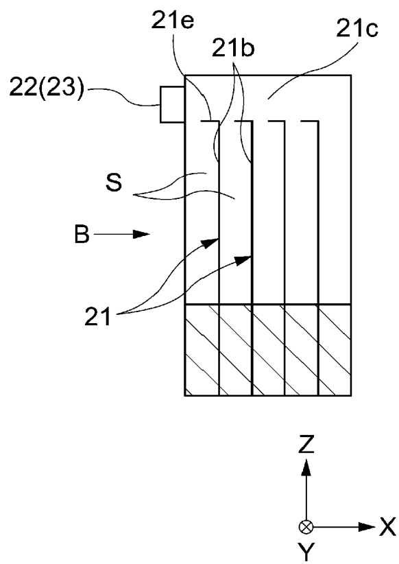
FIG. 9A
