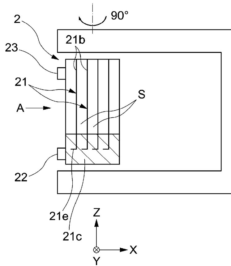
FIG. 8A
